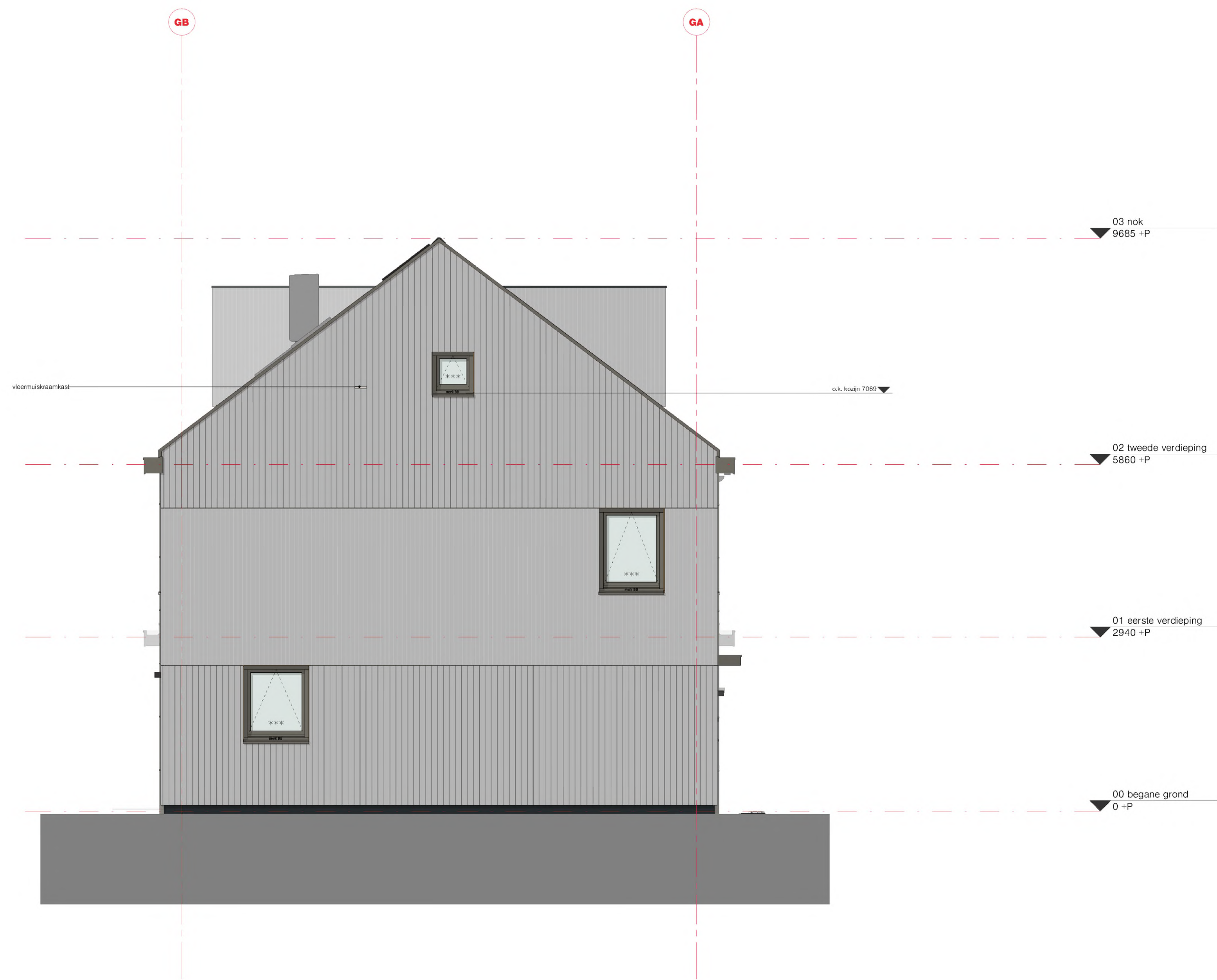
linker zijgevel (L_-_102) schaal: 1 : 50
