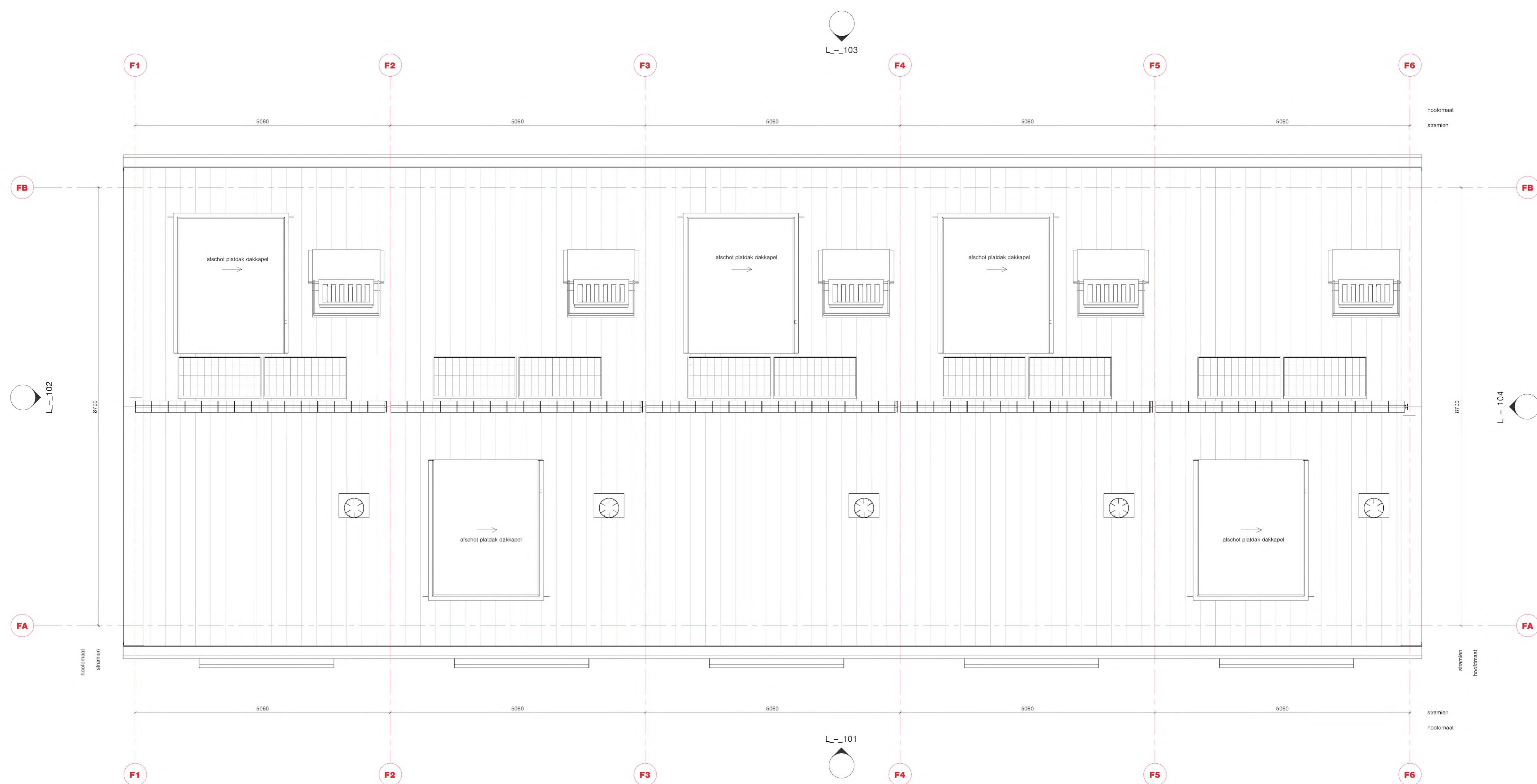
dakaanzicht (L_27_03) schaal: 1 : 50
