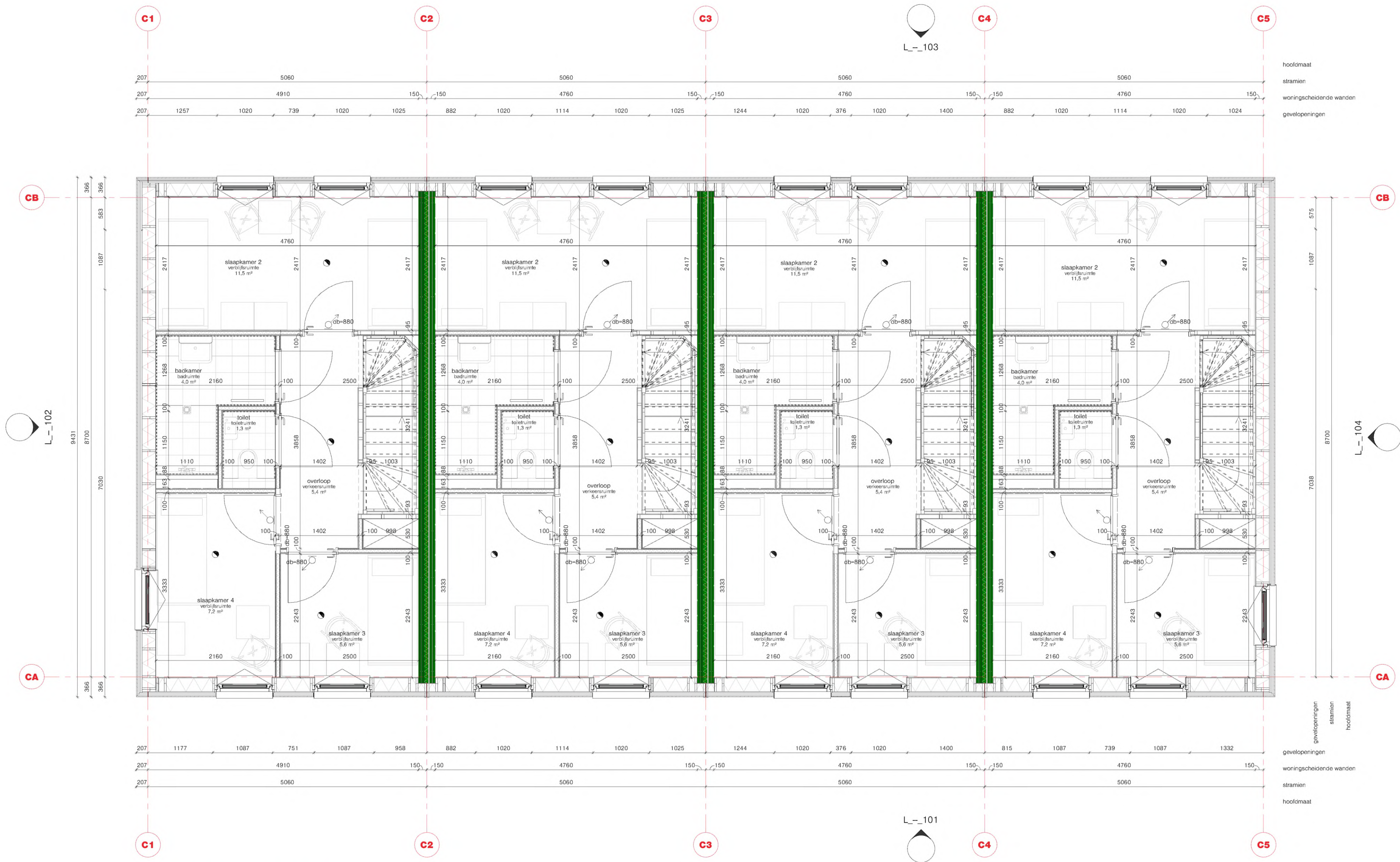
eerste verdieping (L_2_01) schaal: 1 : 50
