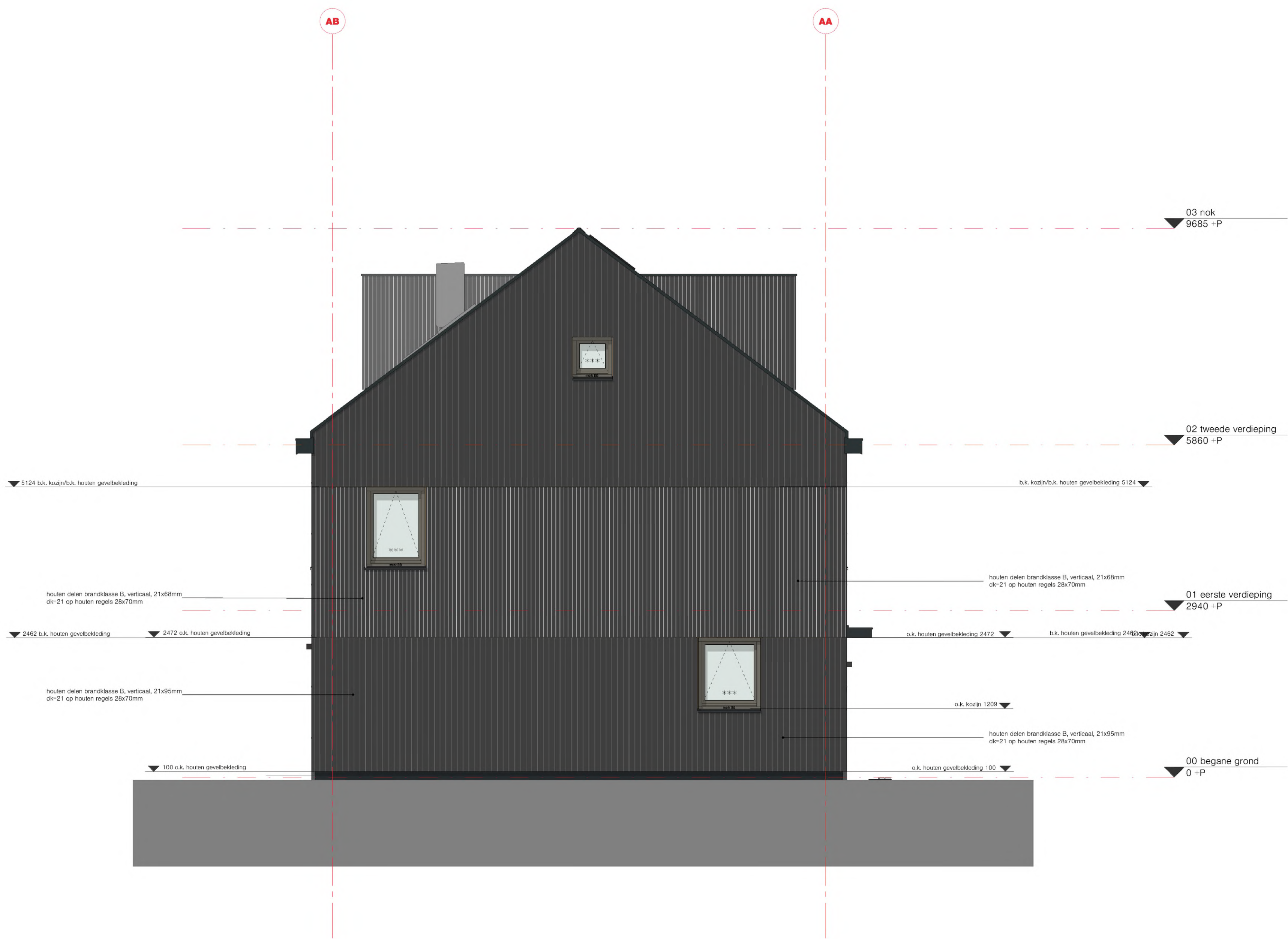
linker zijgevel (L_-_102) schaal: 1 : 50
