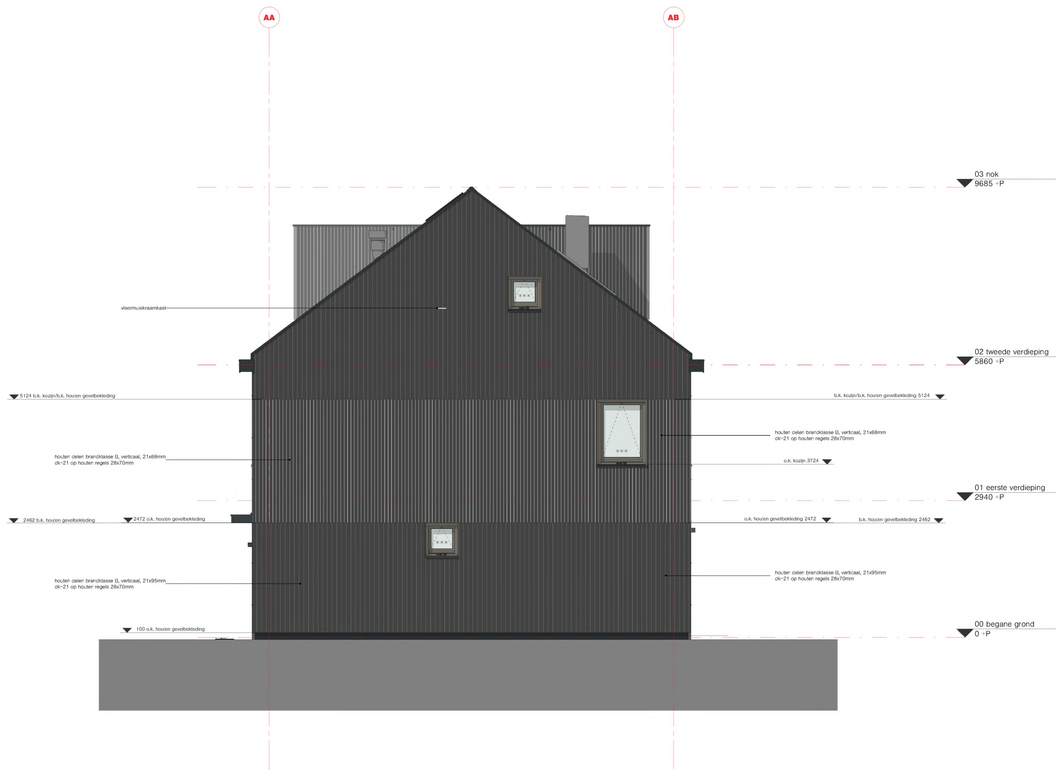
rechter zijgevel (L_-_104) schaal: 1 : 50
