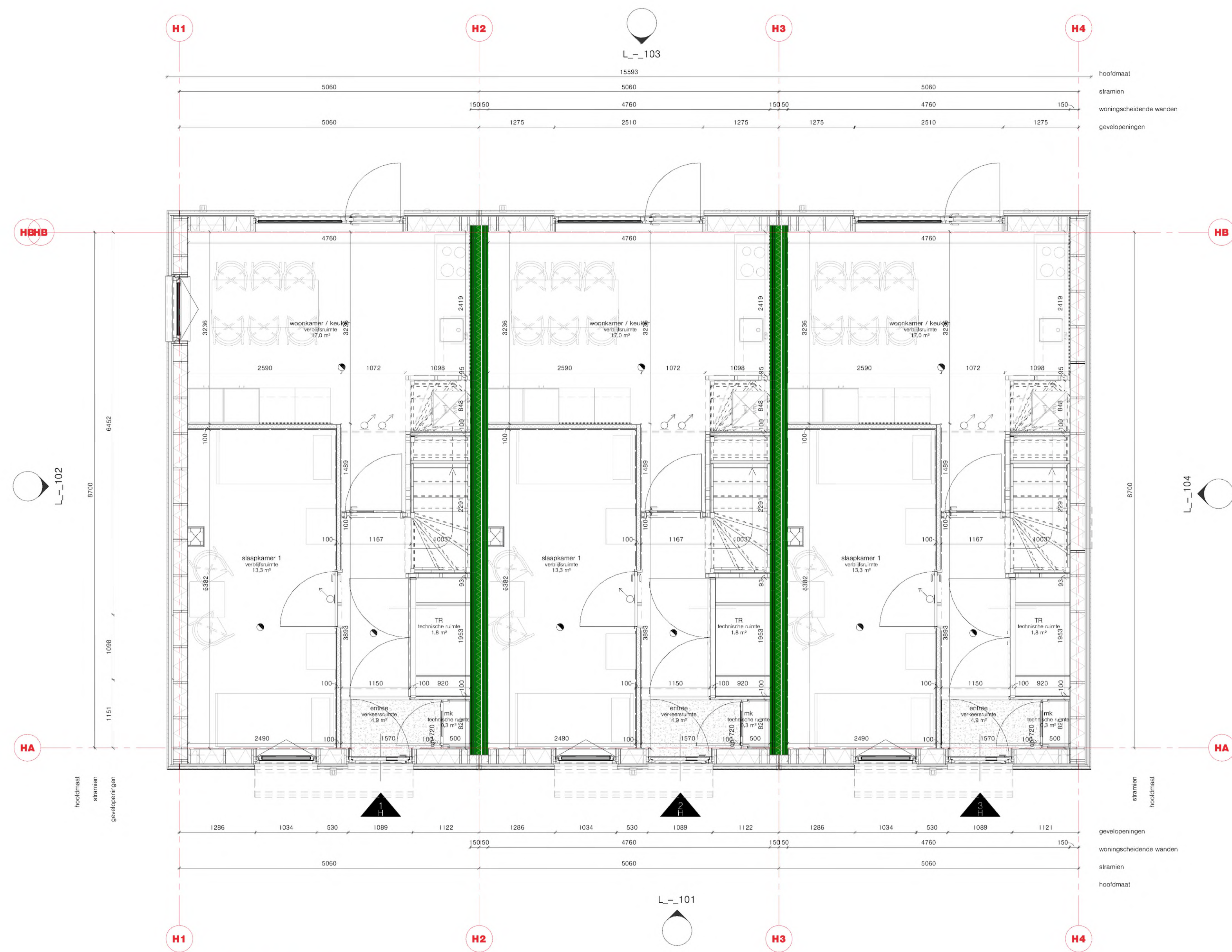
begane grond (L_2_00) schaal: 1 : 50
