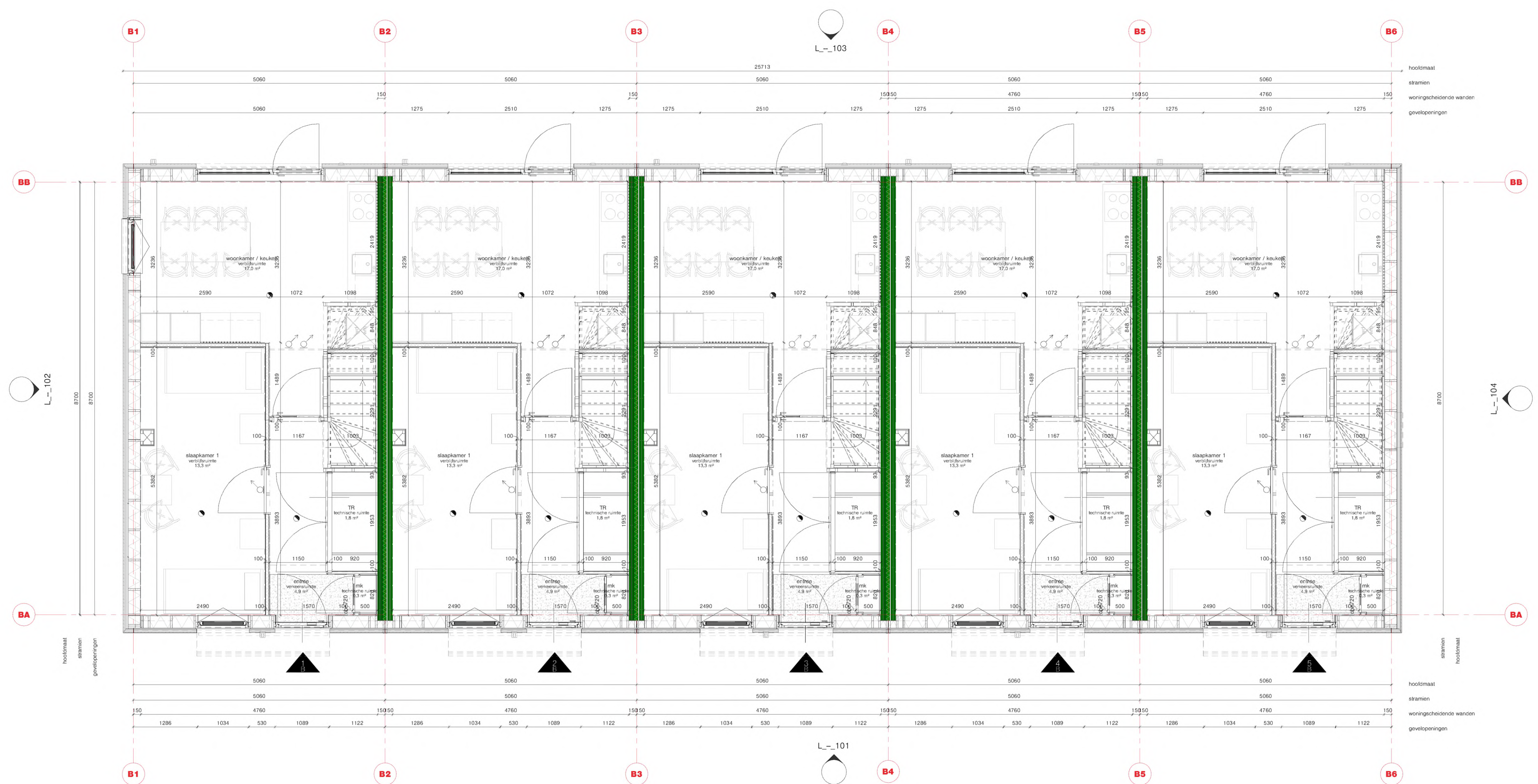
begane grond (L_2-00) schaal: 1 : 50
