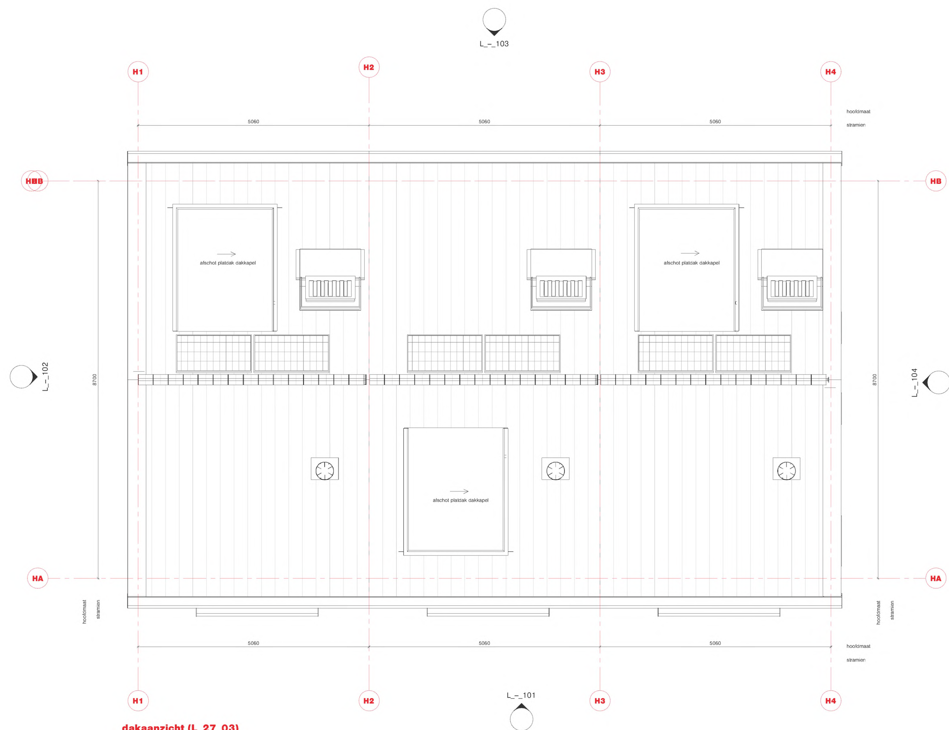
dakaansicht (L_27_03) schaal: 1 : 50
