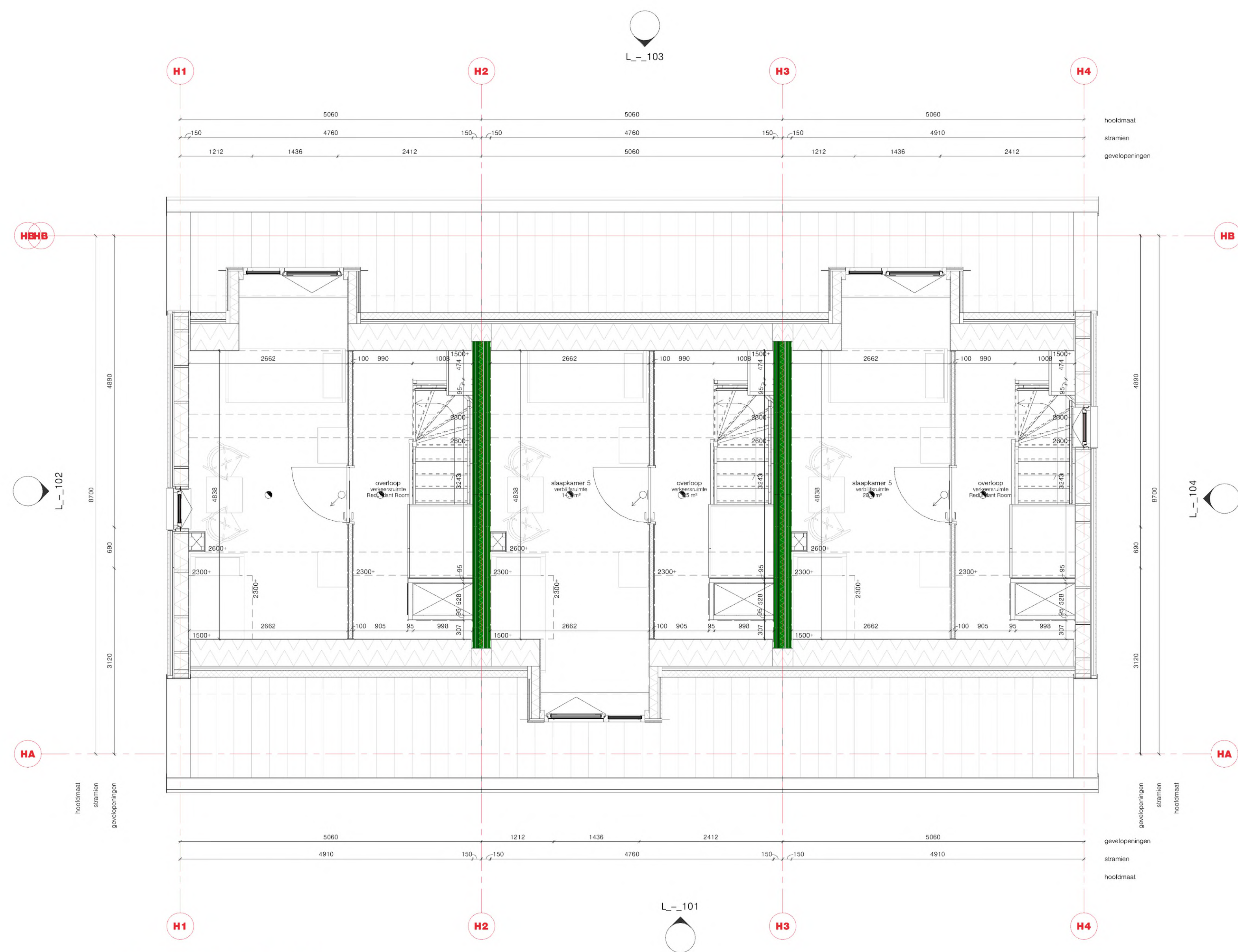
tweede verdieping (L_2_02) schaal: 1 : 50
