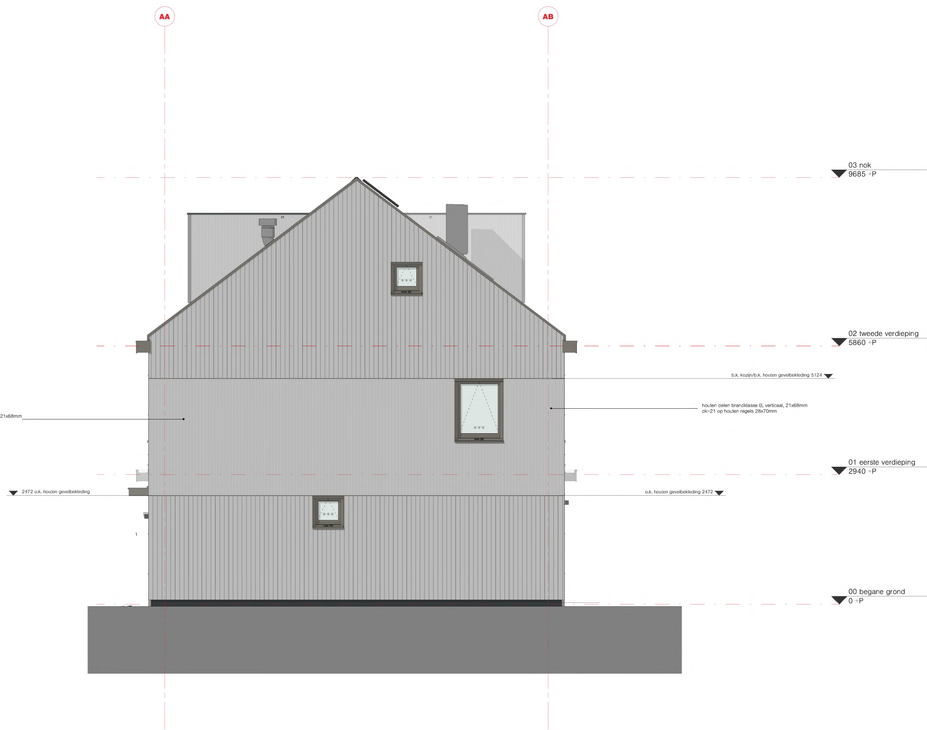
rechter zijgevel (L_-_104) schaal: 1 : 50
