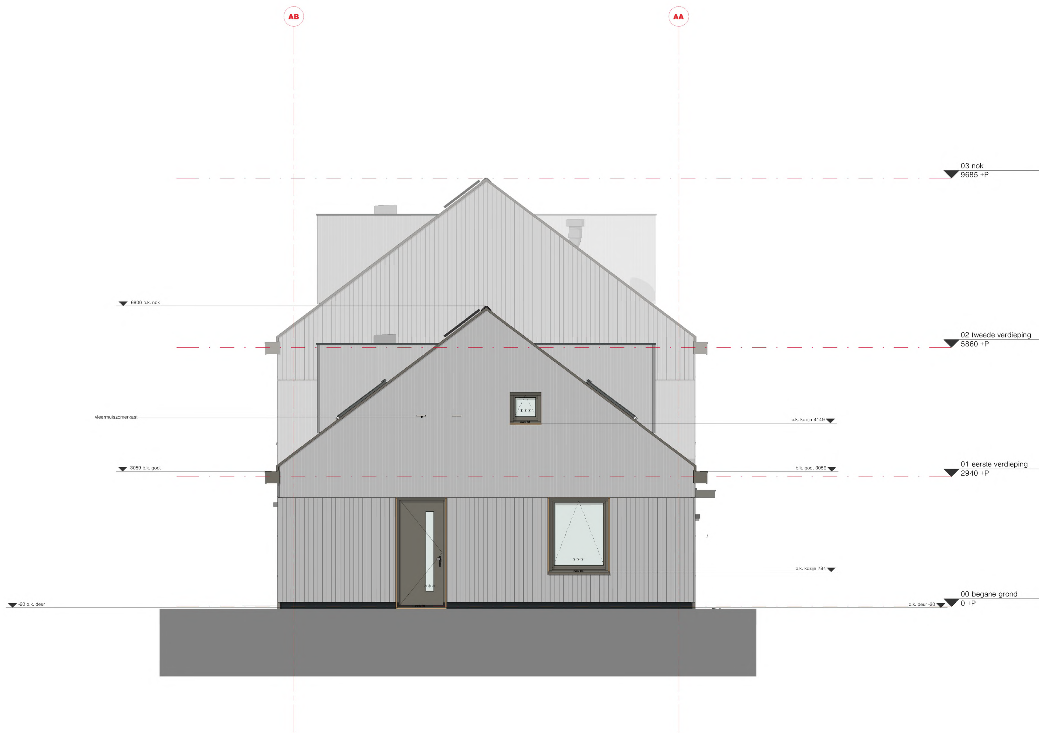
linker zijgevel (L_-_102) schaal: 1 : 50
