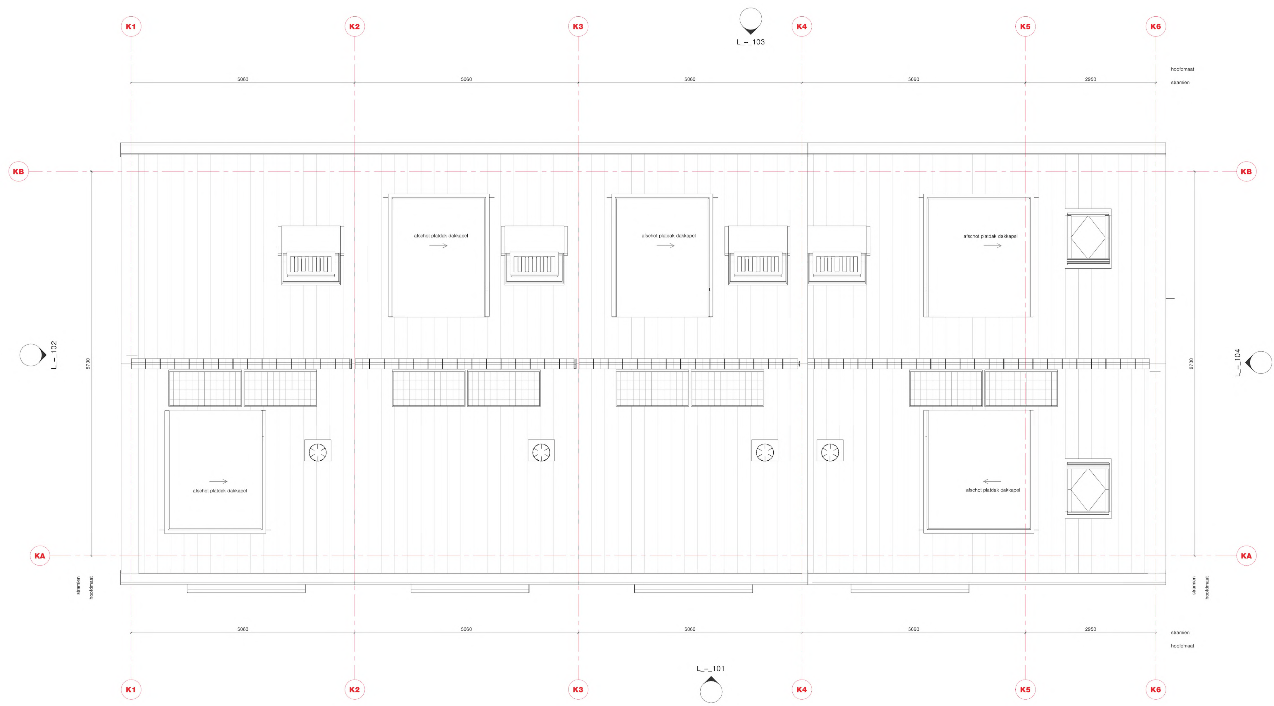
dakaanzicht (L_27_03) schaal: 1 : 50
