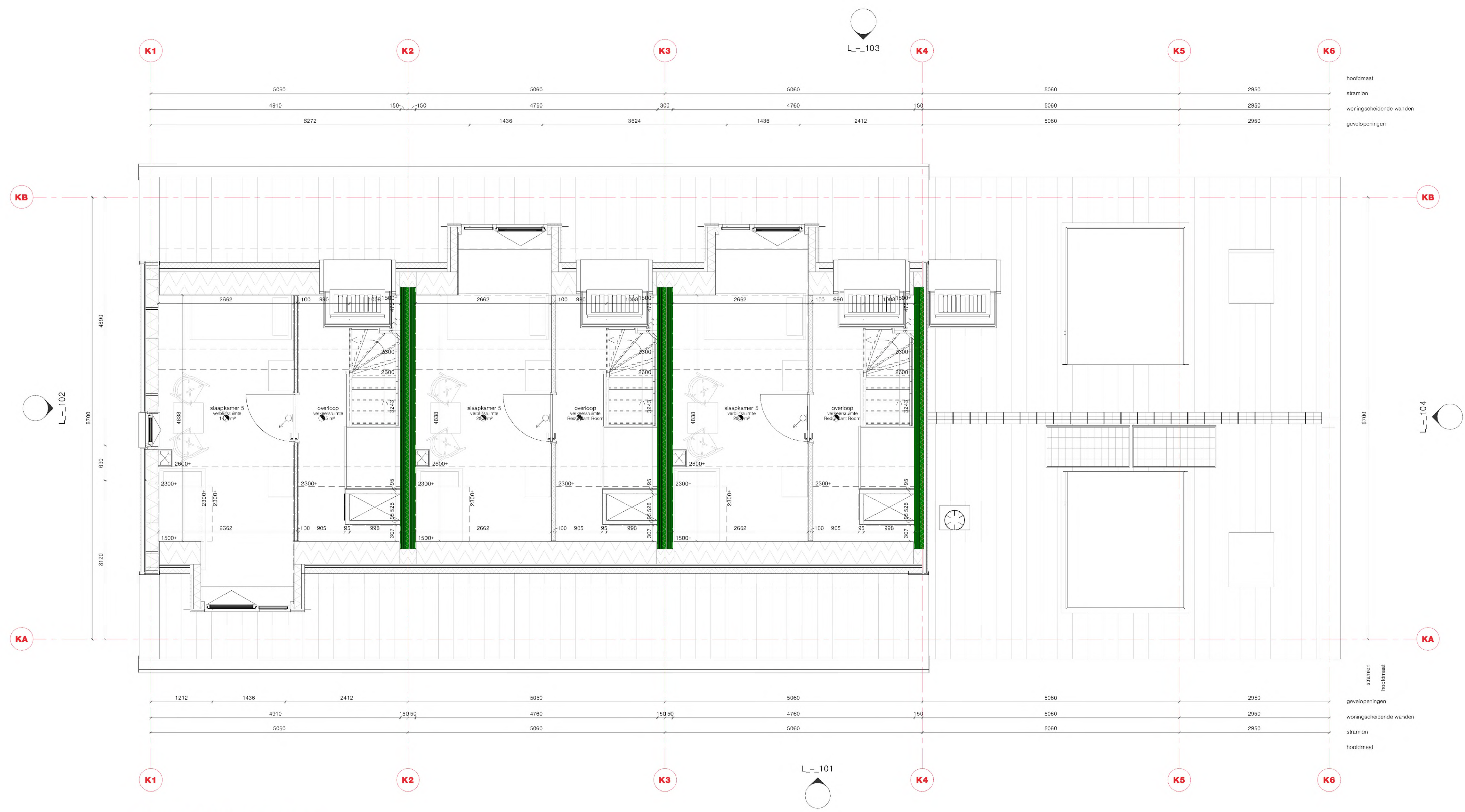
tweede verdieping (L_2_02) schaal: 1 : 50
