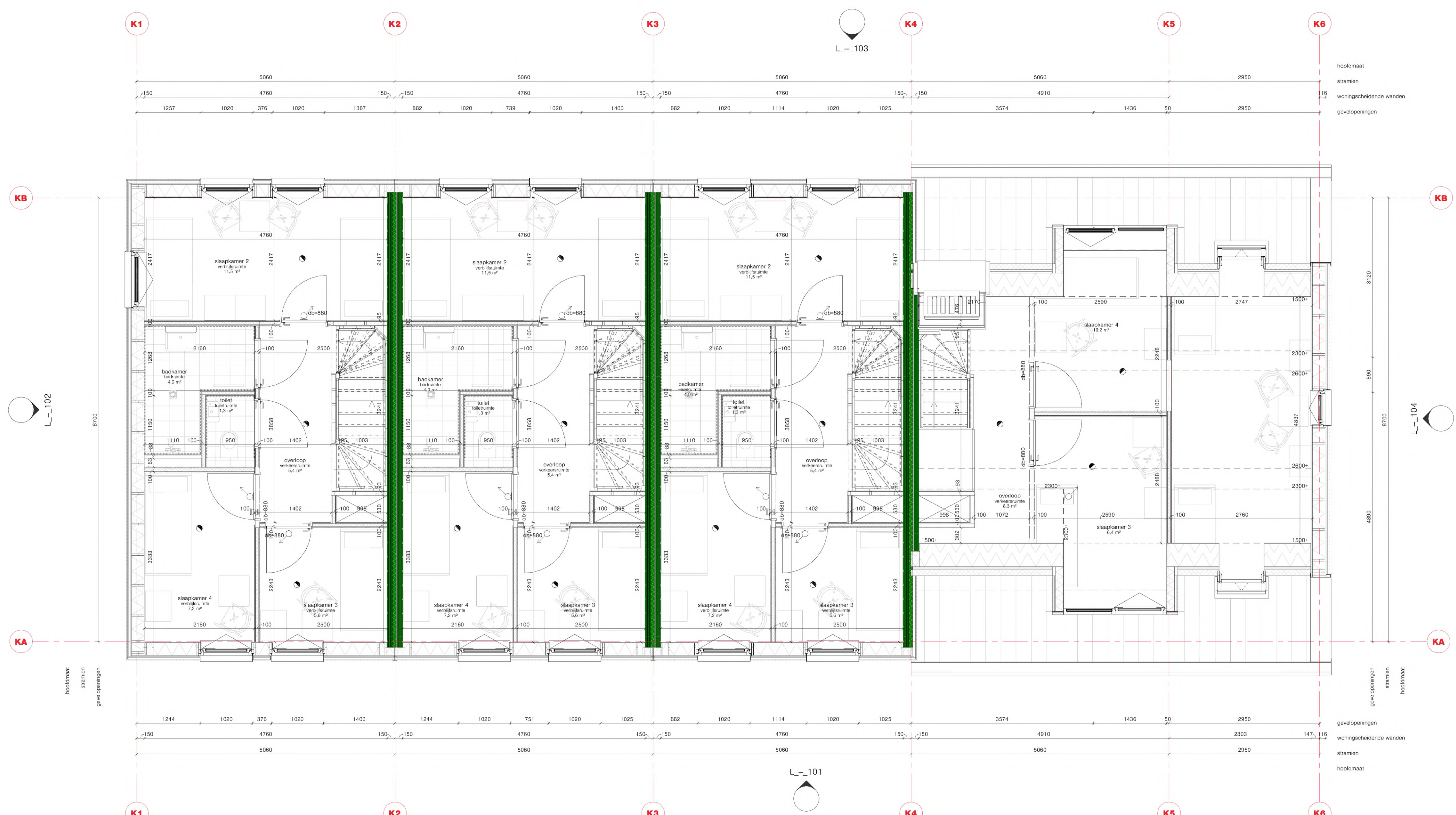
eerste verdieping (L_2_01) schaal: 1 : 50
