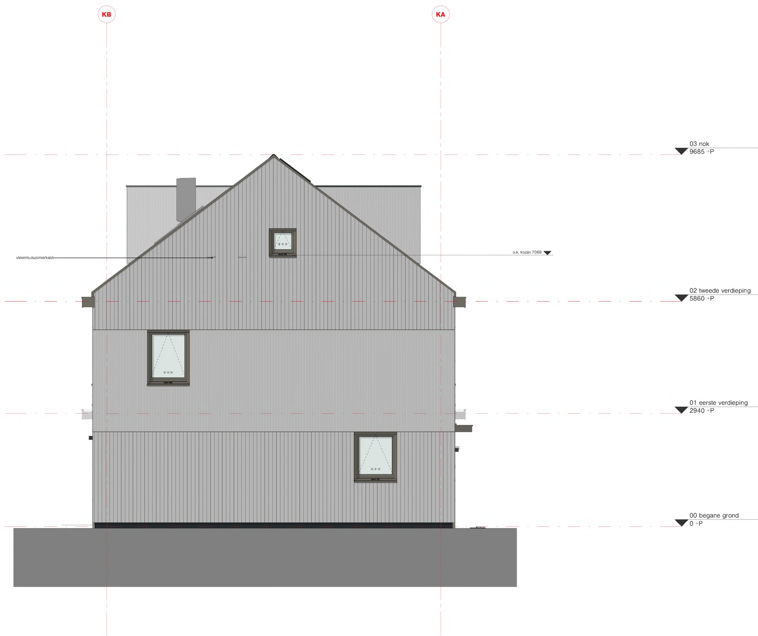
linker zijgevel (L_-_102) schaal: 1 : 50
