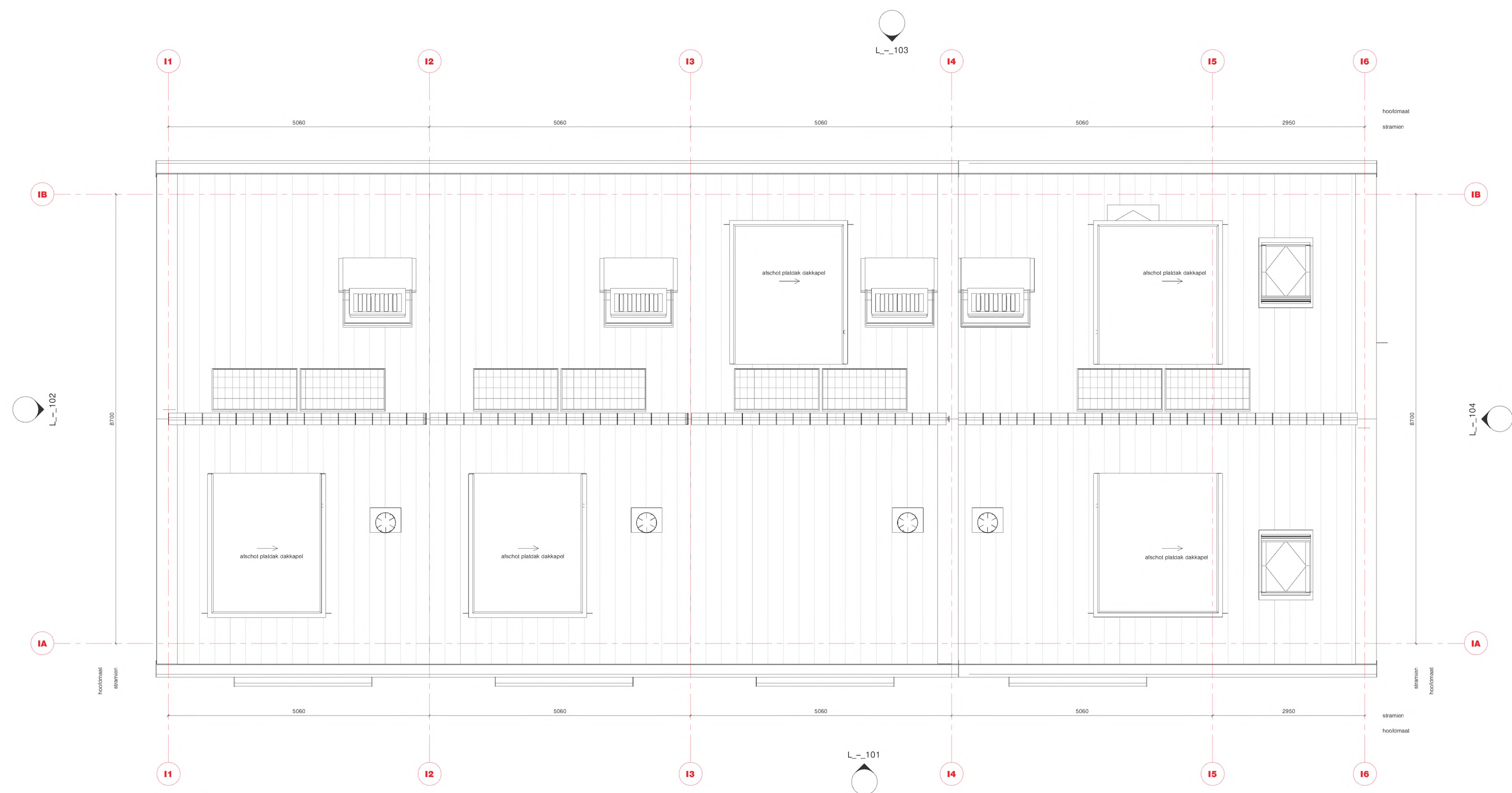
dakaansicht (L_27_03) schale: 1 : 50
