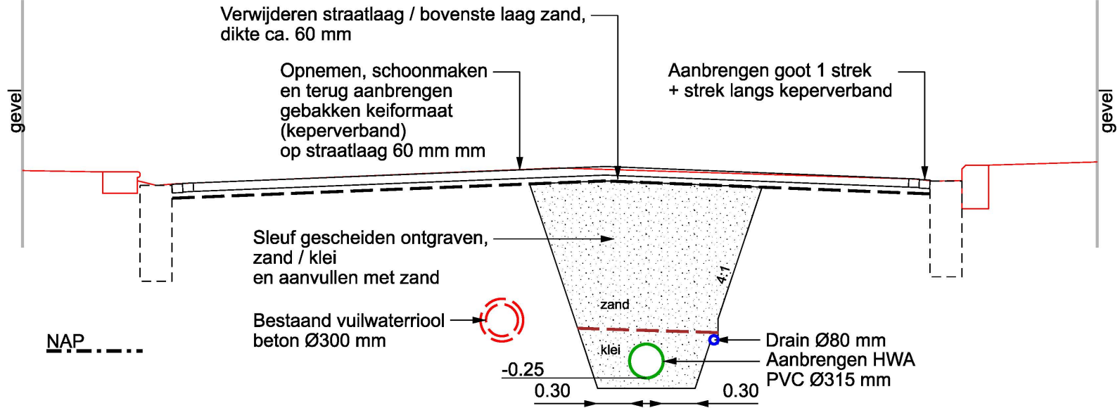
PROFIEL F-F schaal 1:50
