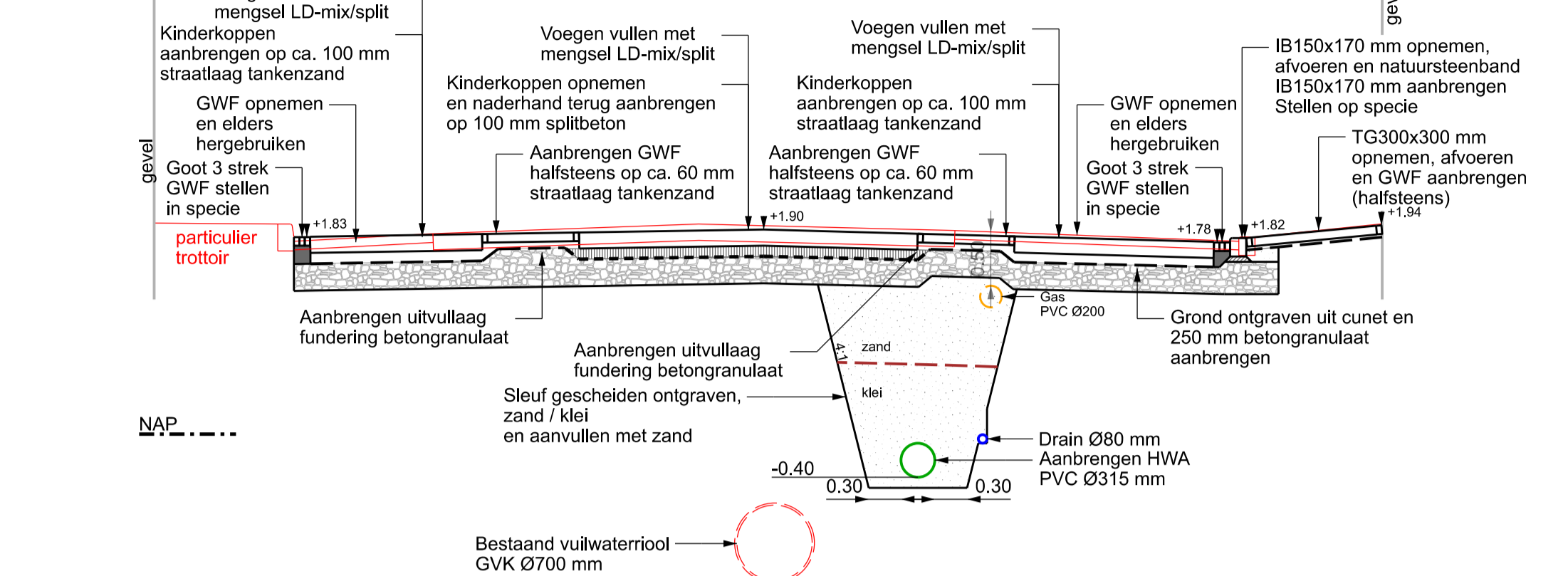
PROFIEL D-D schaal 1:50
