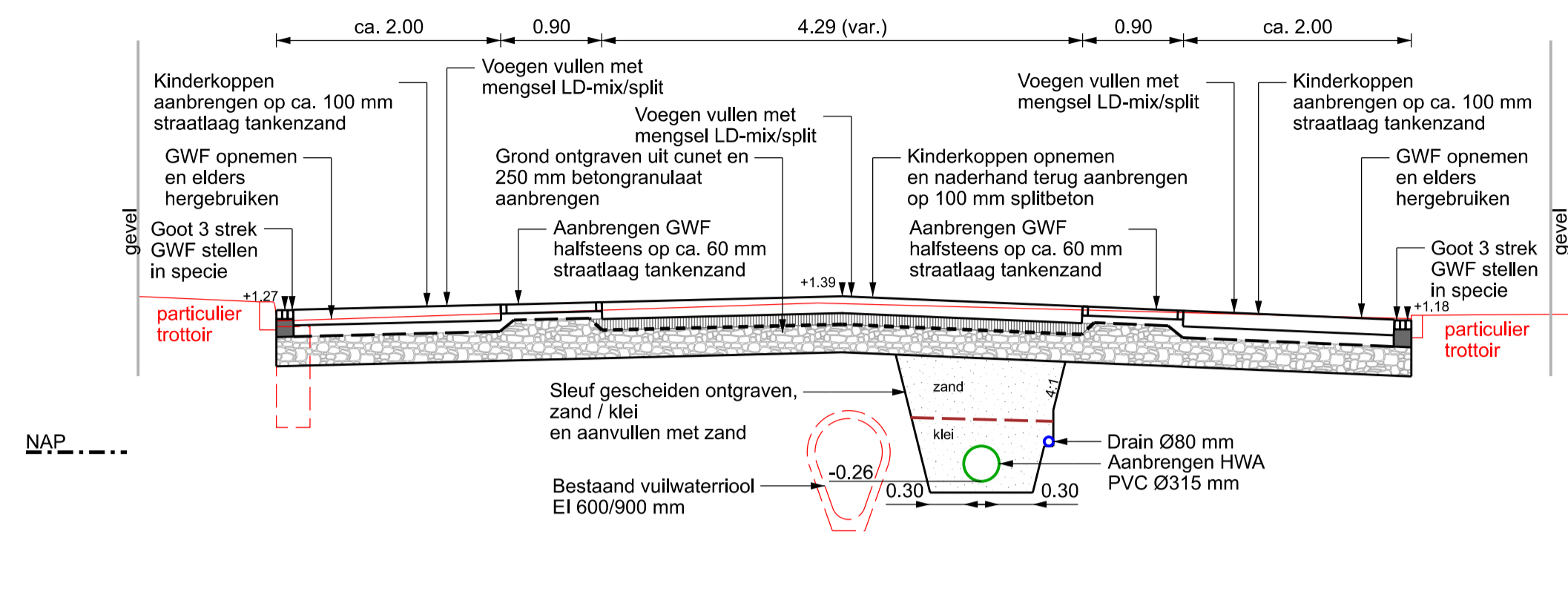
PROFIEL A-A schaal 1:50
