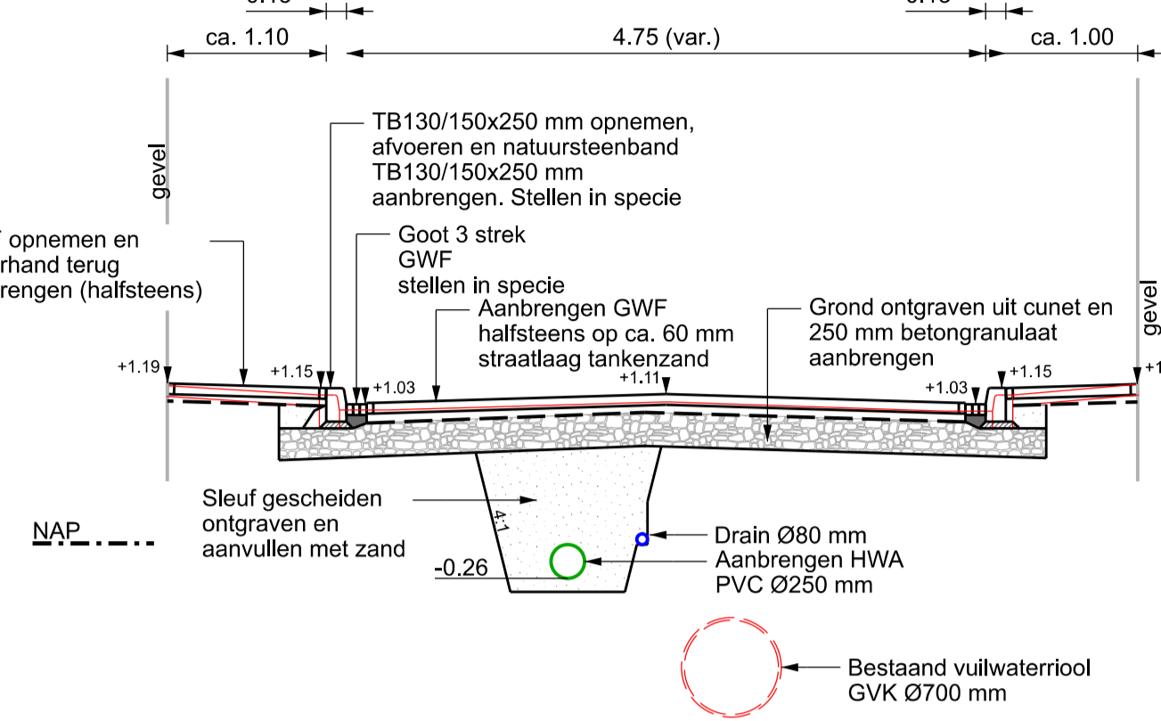
PROFIEL B-B schaal 1:50
