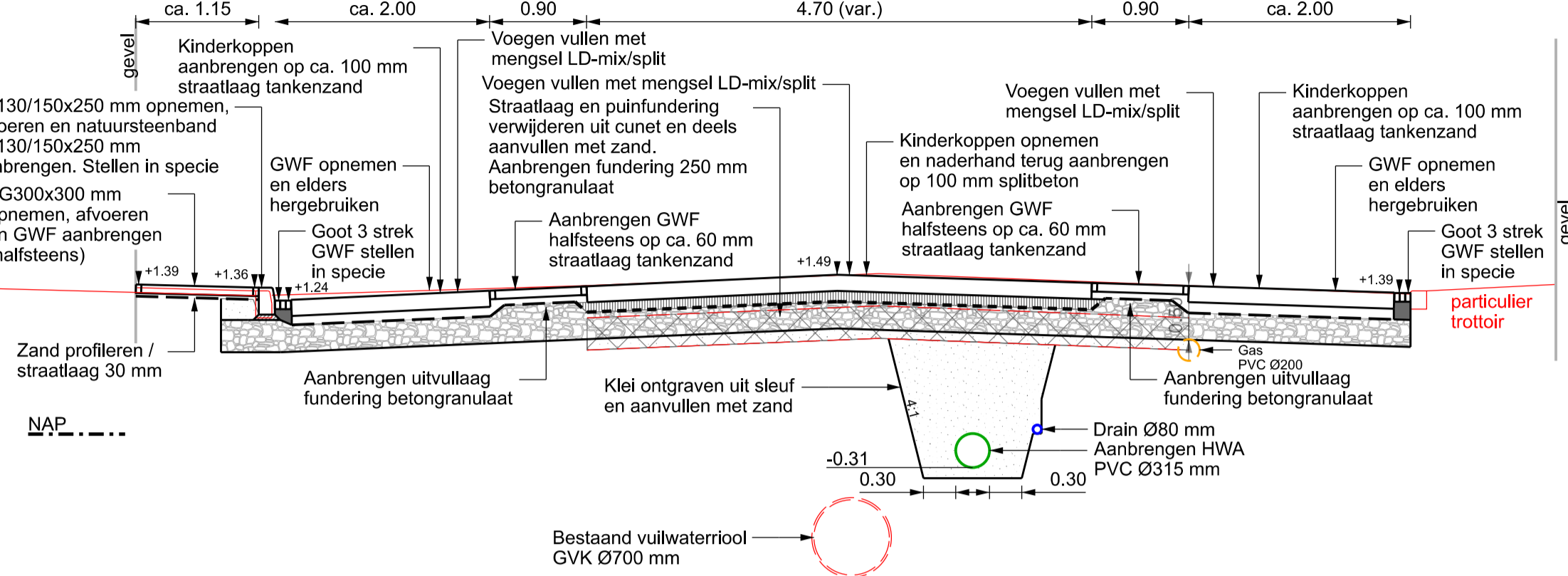
PROFIEL C-C schaal 1:50
