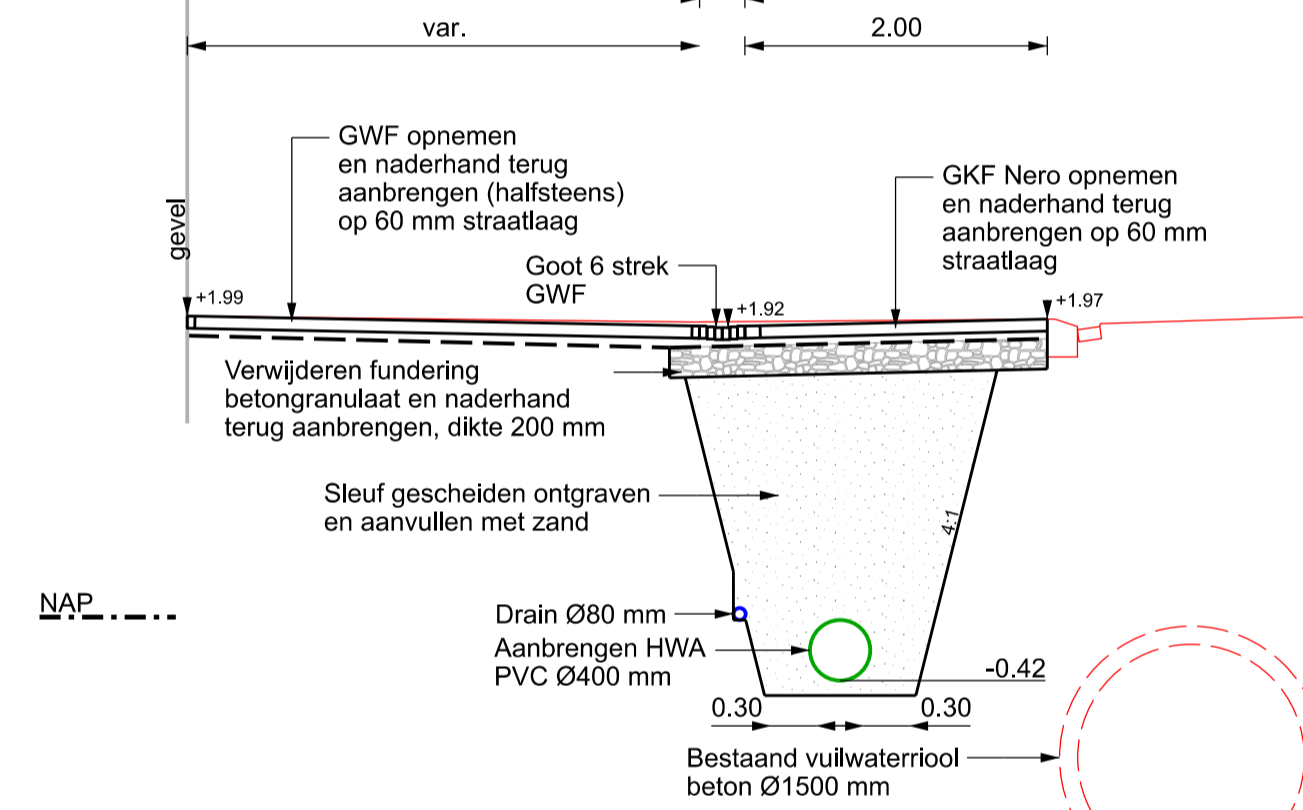
PROFIEL E-E schaal 1:50
