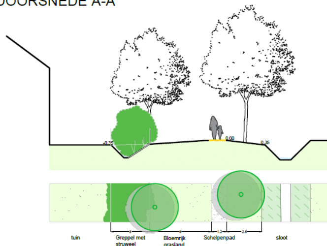
DOORSNEDE A-A'
