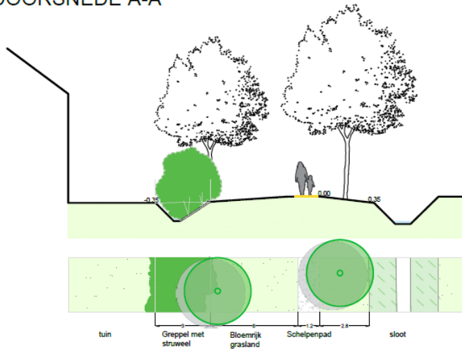
DOORSNEDE A-A'
