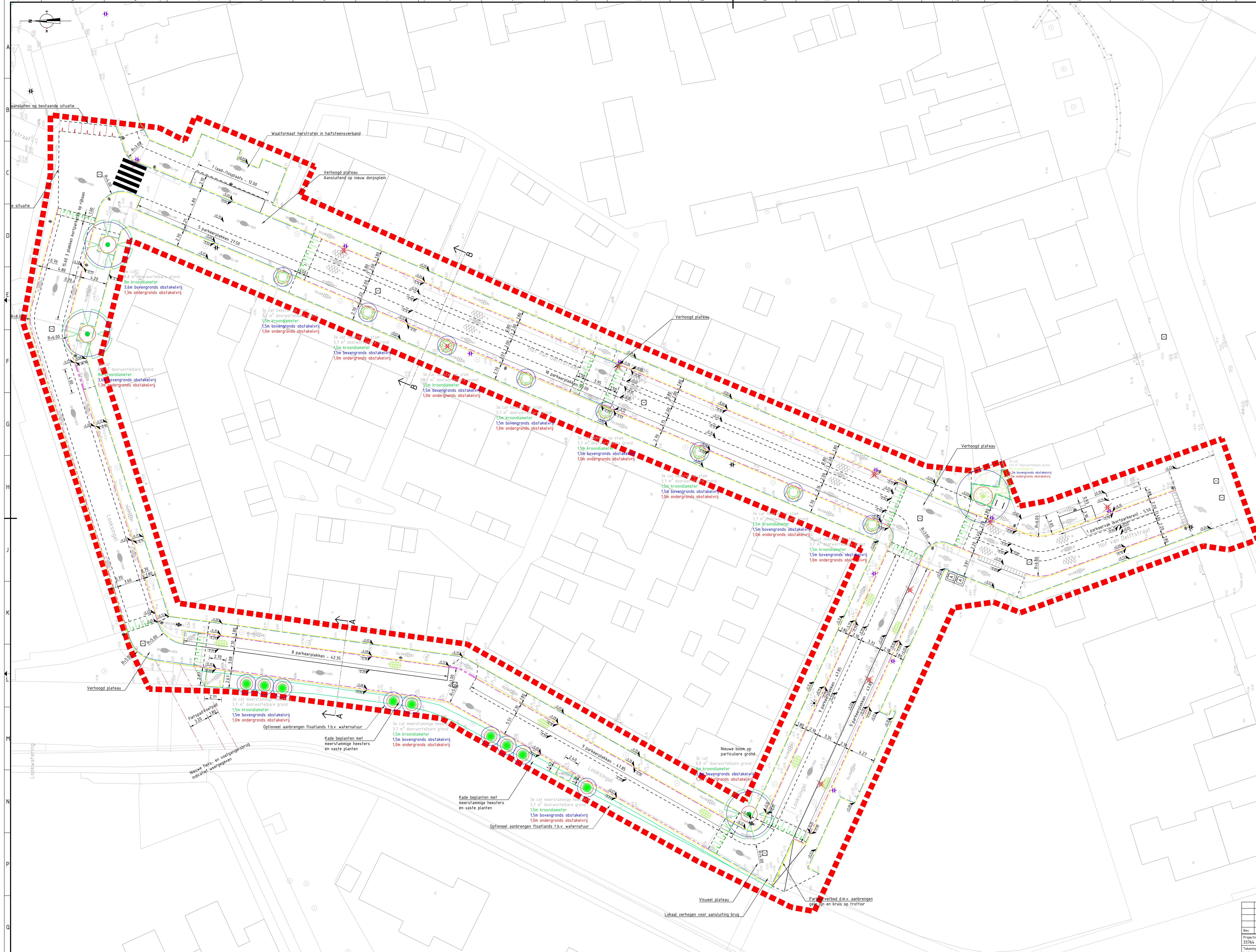
Bovenaanzicht 1 SCHAAL 1 : 200
