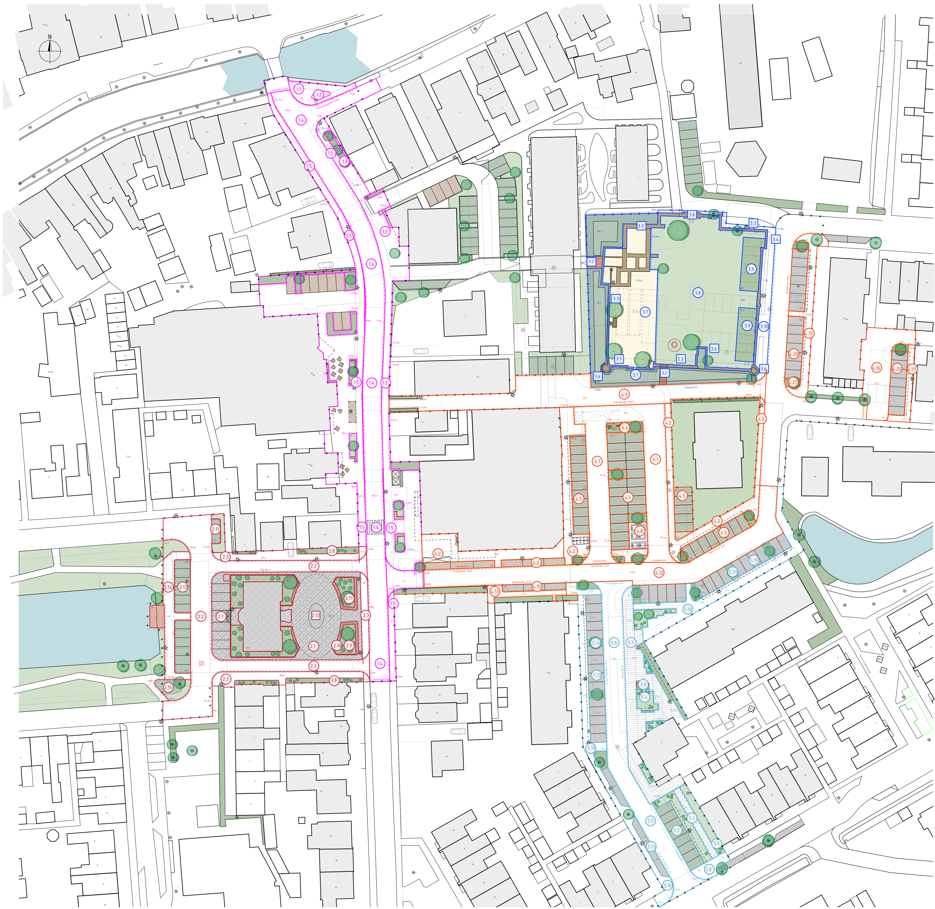
SITUATIE SCHAAL 1:500
