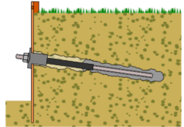
Schematische weergave van een groutanker
