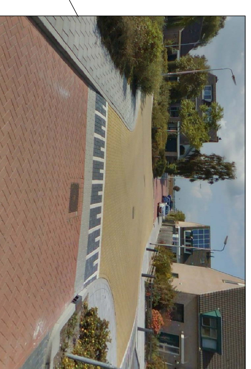
Drempelplateau op gelijkwaardig kruispunt
