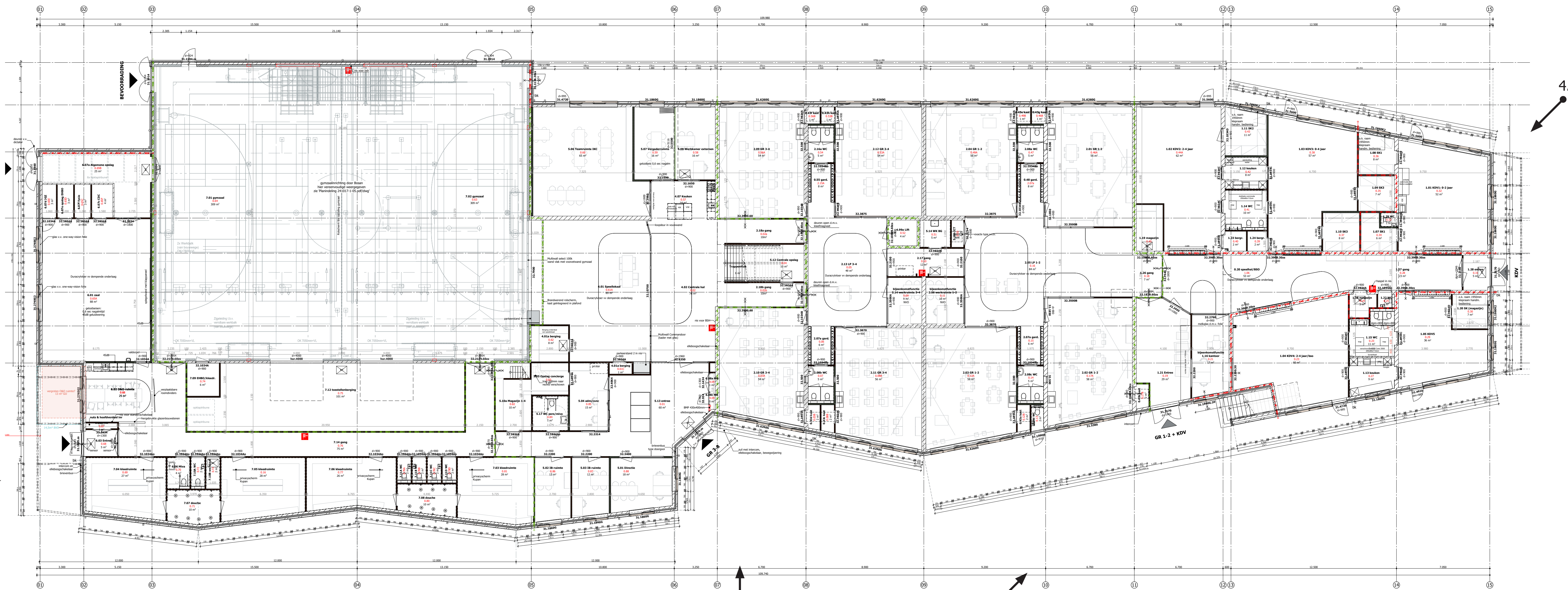
plattegrond | begane grond
