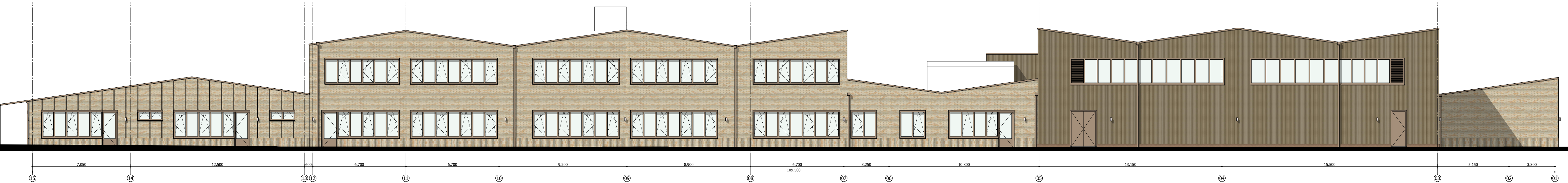
noordgevel | klaslokalen en gymzaal
