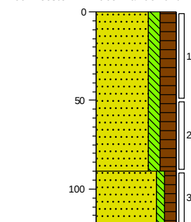
Boring: 2 Datum: 31-1-2023 Boormeester: Ruben van de Bunt
