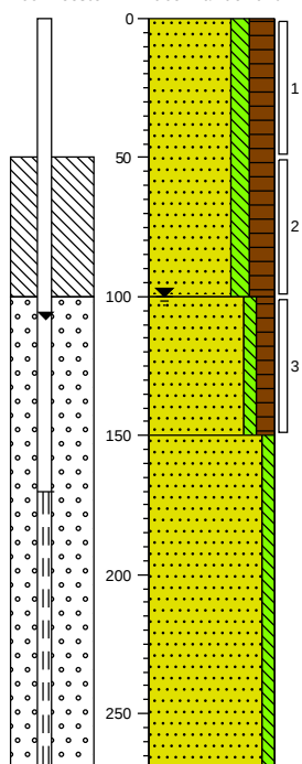
Boring: 1 Datum: 31-1-2023 Boormeester: Ruben van de Bunt
