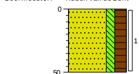
Boring: 5 Datum: 31-1-2023 Boormeester: Ruben van de Bunt
