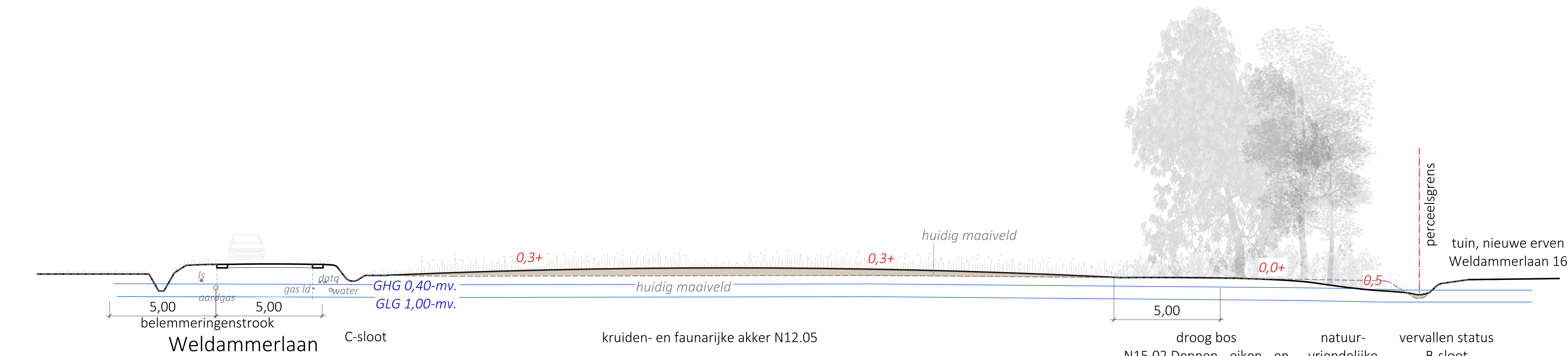
PROFIEL M-M' schaal 1:100
