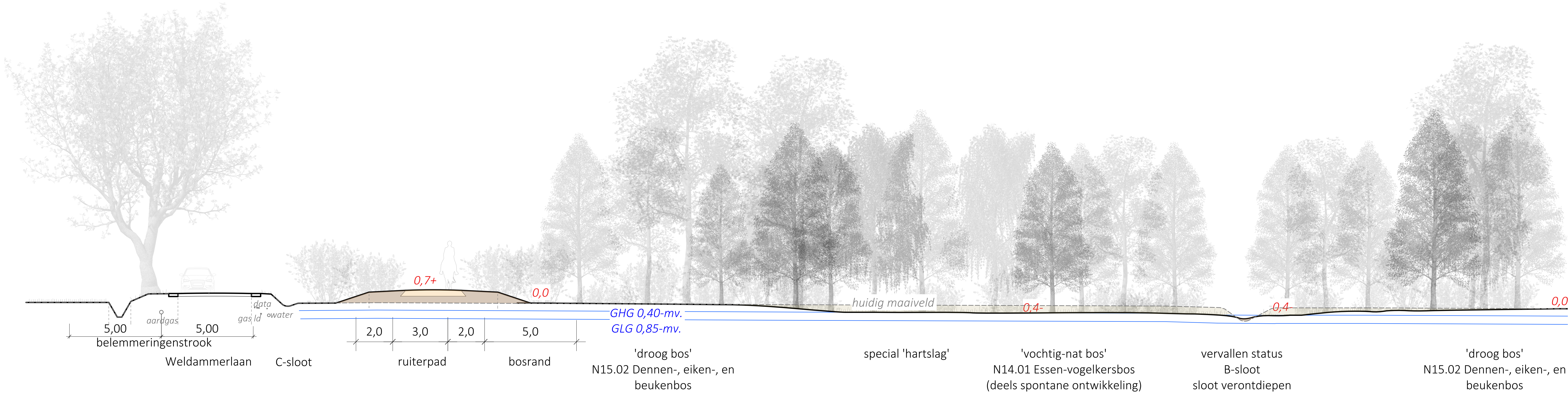
PROFIEL NO-NO' schaal 1:100
