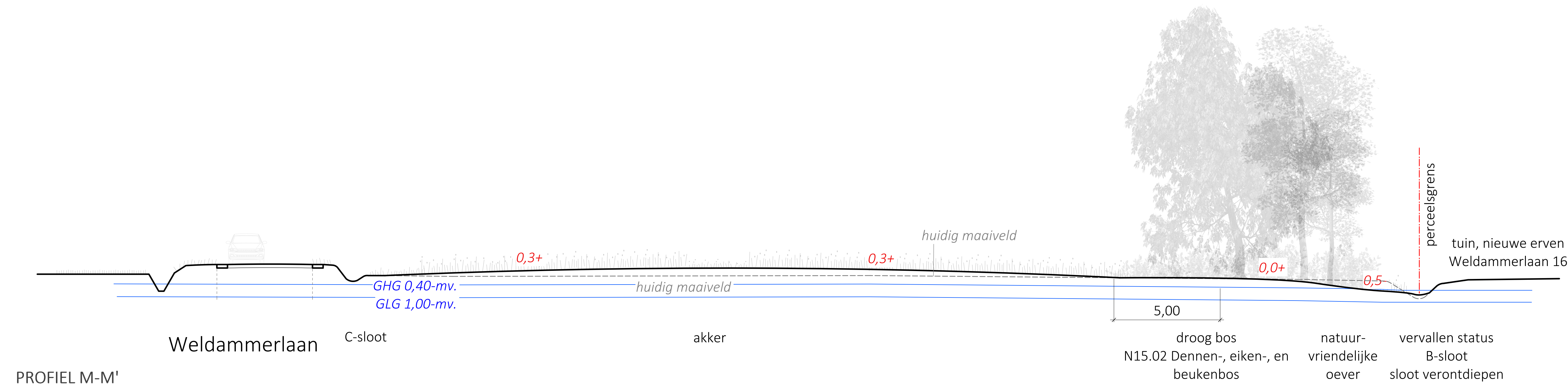
PROFIEL M-M' schaal 1:100
