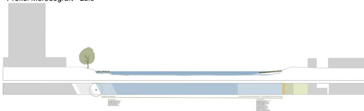
Profiel Merodegraft - zuid
