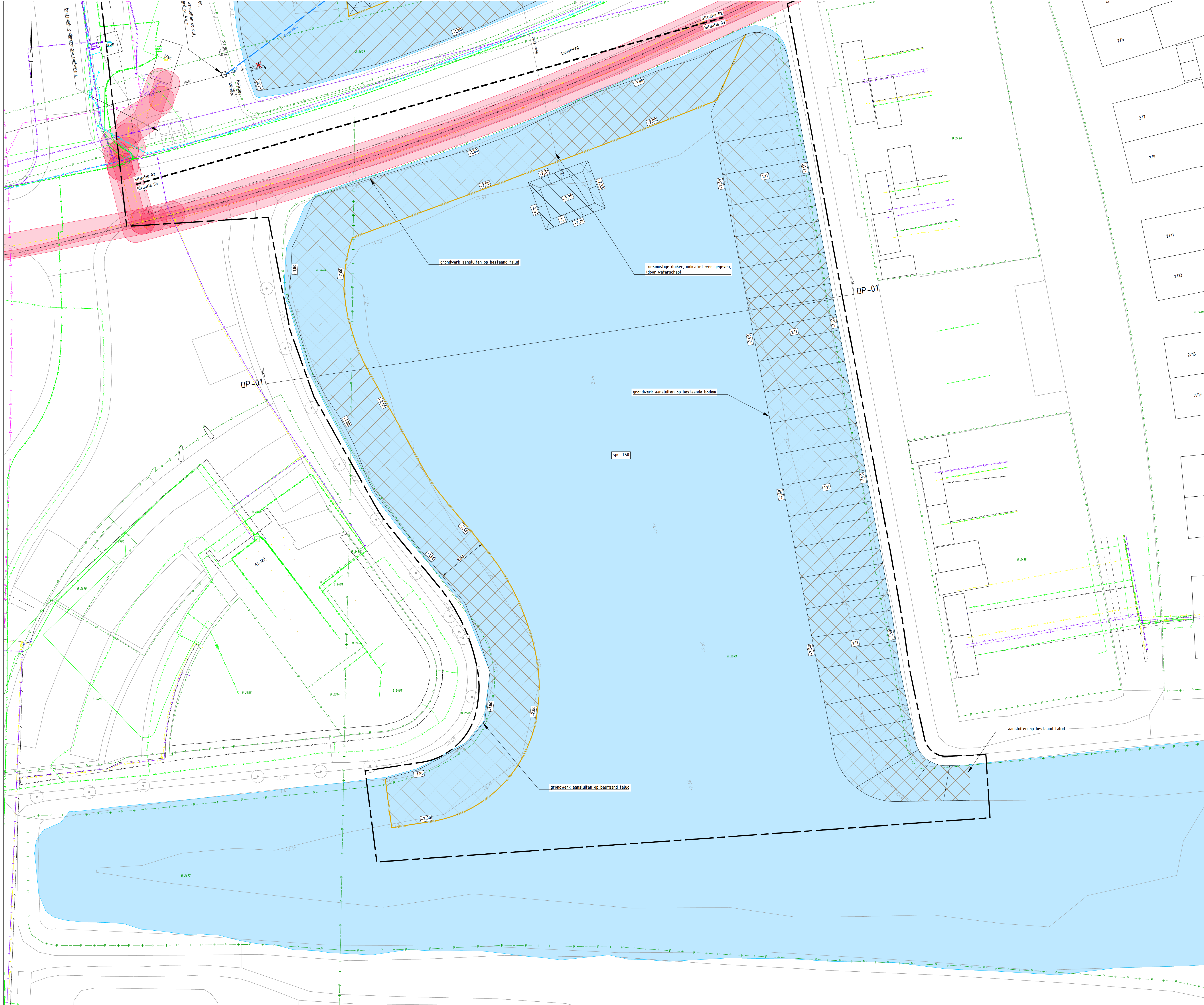
SITUATIE 03 schaal 1:200
