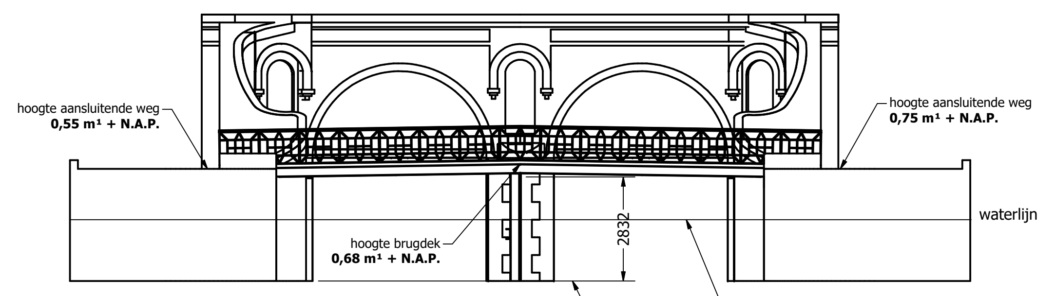
Aanzicht zuidzijde
