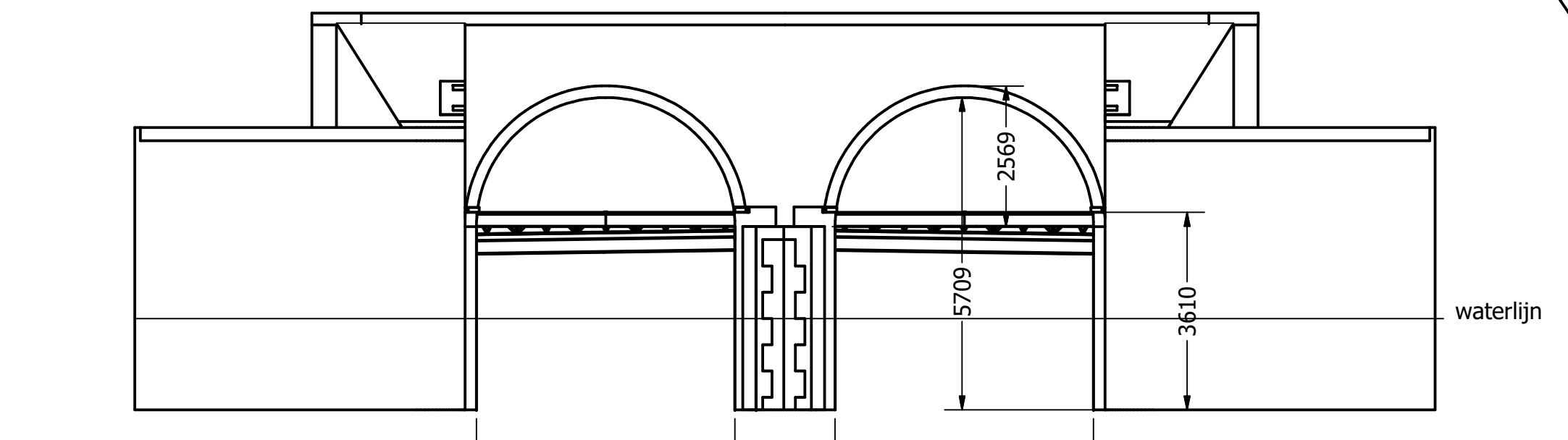
Aanzicht noordzijde
