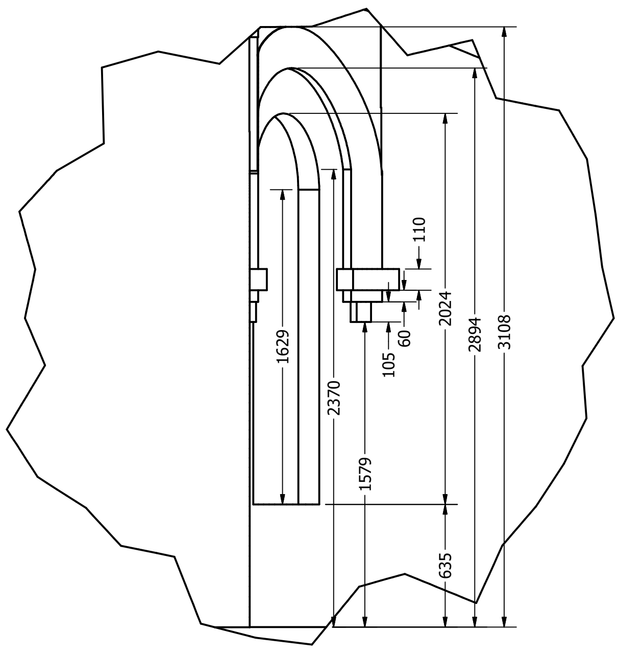
DETAIL E SCALE 1 / 20 zijnissen
