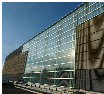
Figuur 8: zonnepanelen in geluidsscherm © TNO
