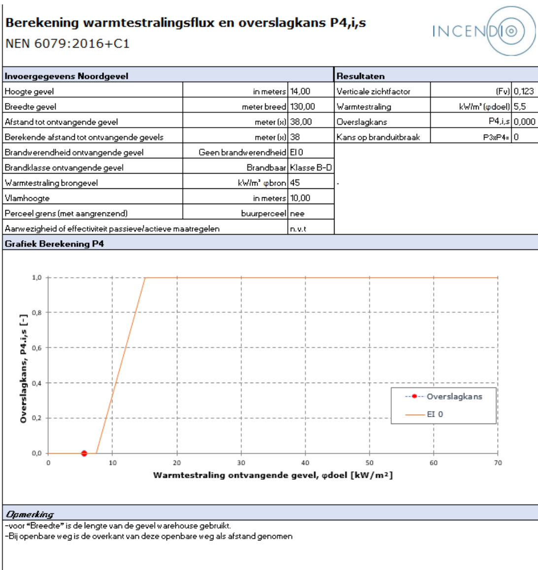
Figuur 11 Berekening van de noordgevel
