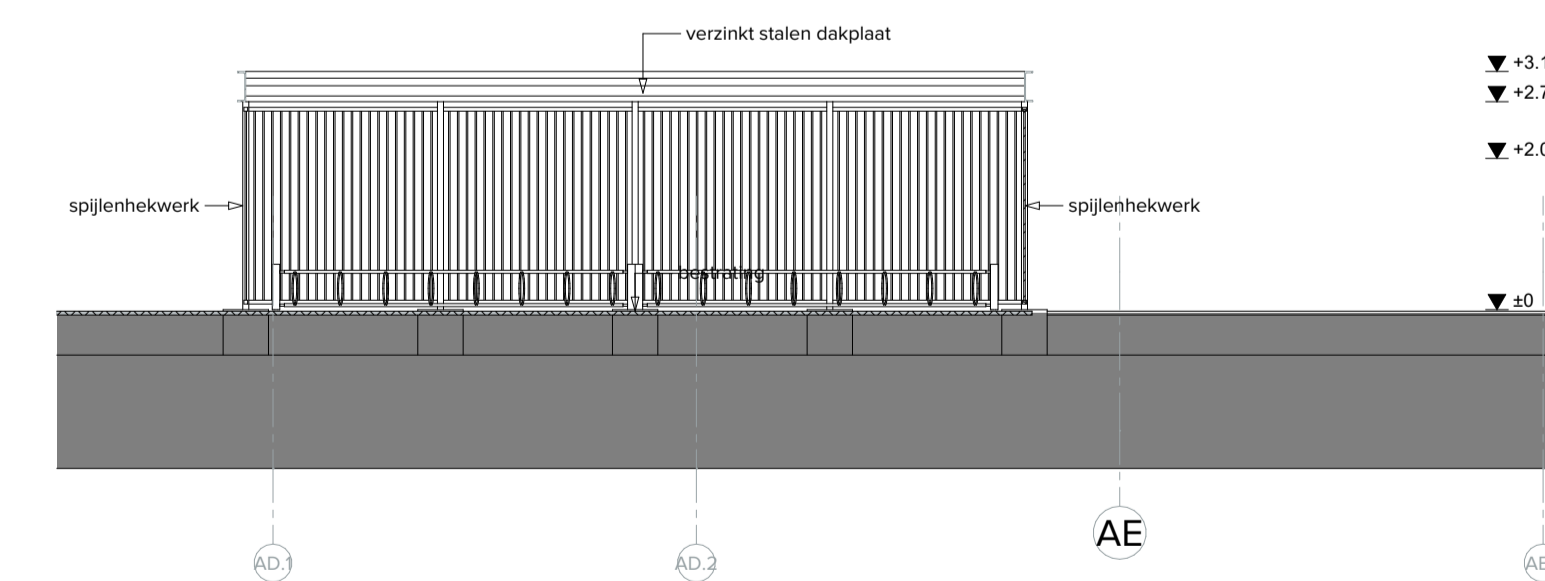
Doorsnede A Fietsenstalling
