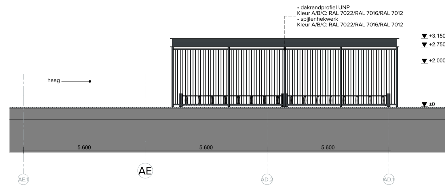
Linkergevel Fietsenstalling
