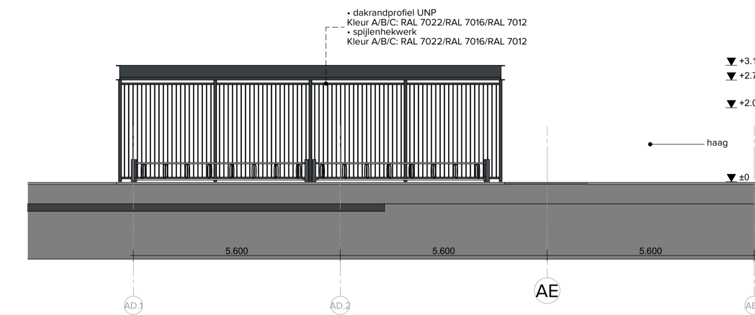
Rechtergevel Fietsenstalling
