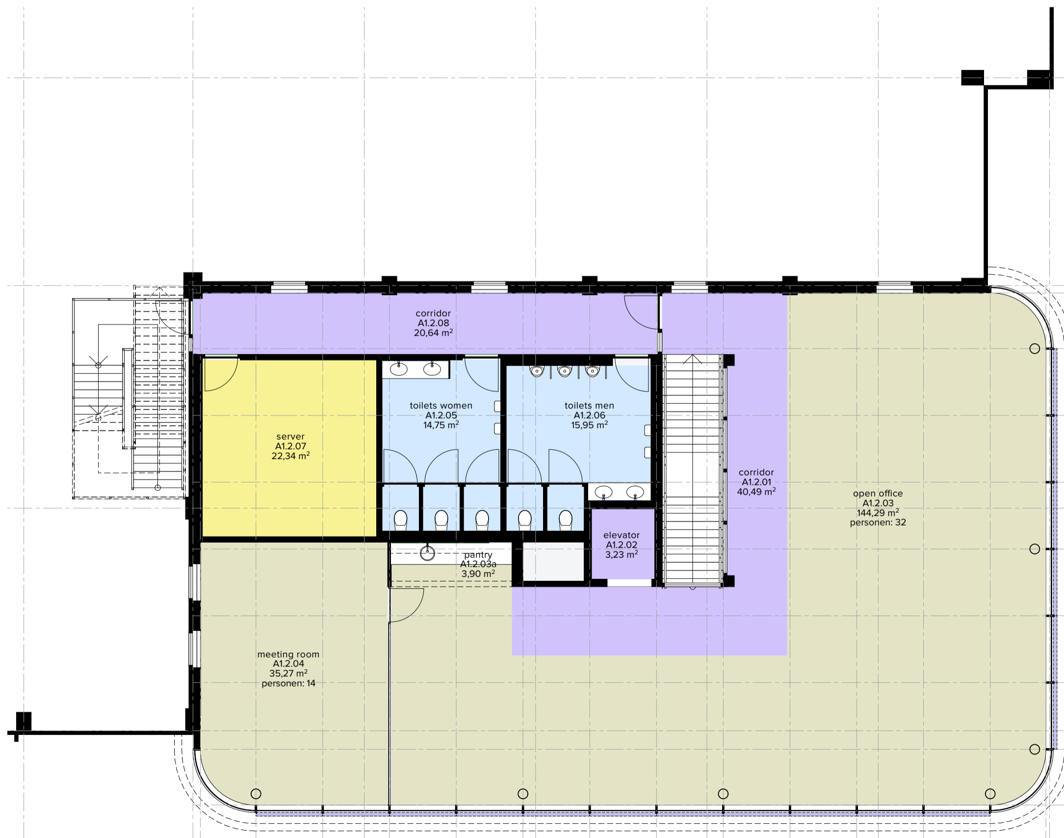
2e verdieping
