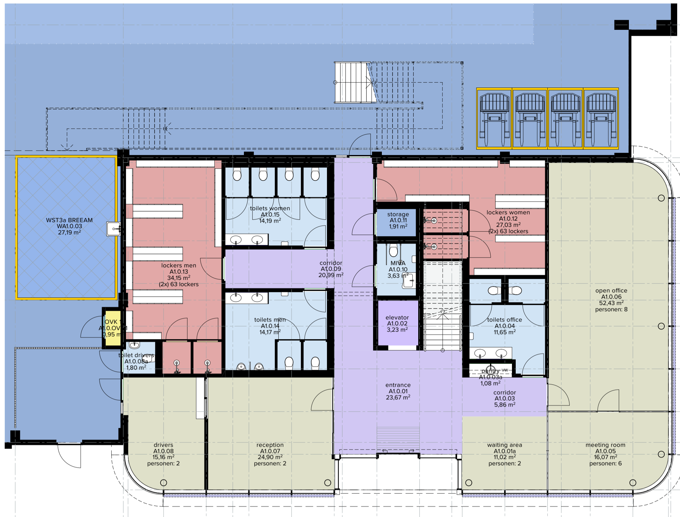
begane grond
