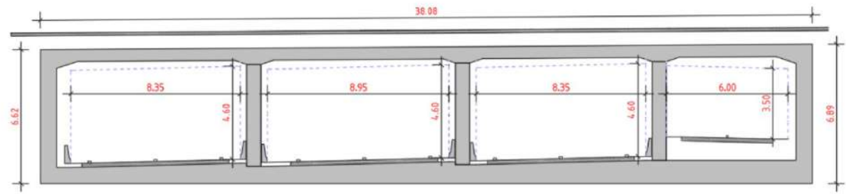
afbeelding : weergave doorsnede nieuwe tunnel onder de A58
