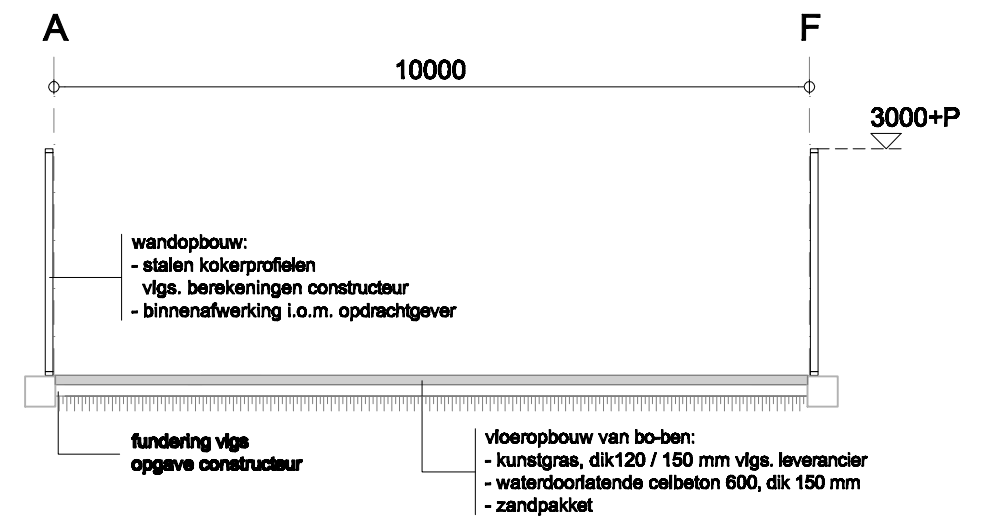
DOORSNEDE
