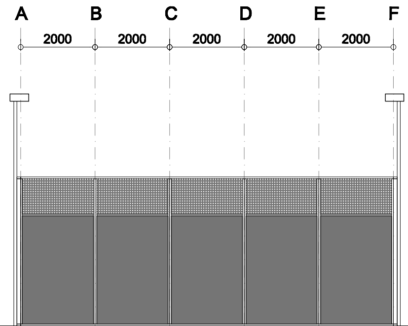
ZIJAAANZICHT
