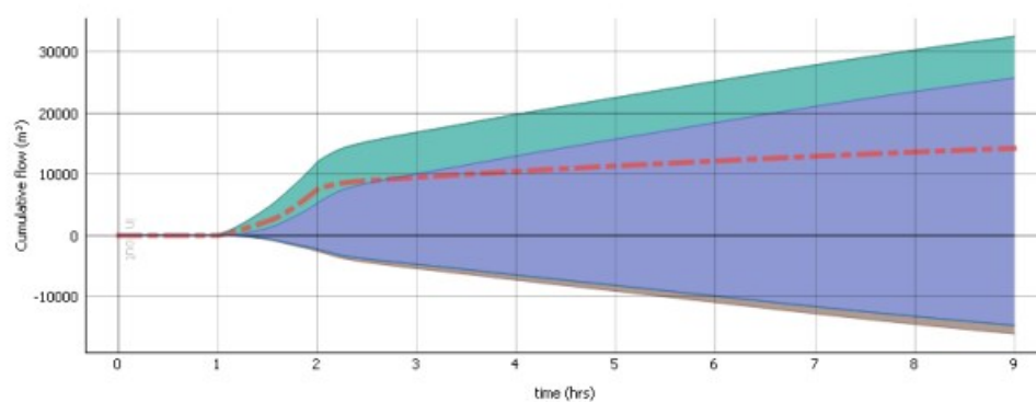
Figuur 4-4 Cumulatieve waterbalans toekomst situatie in T100-scenario
