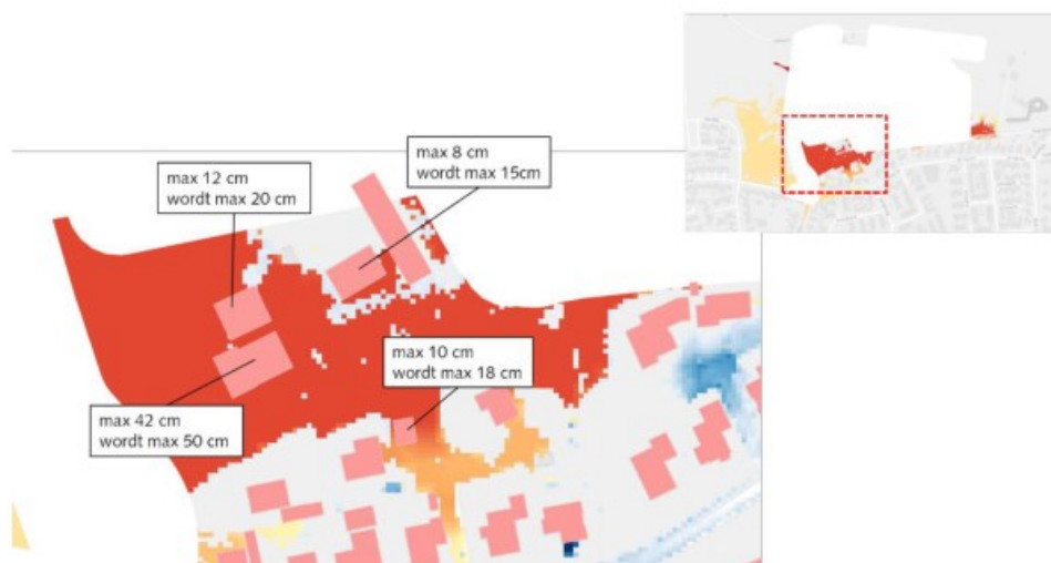
Figuur 4-5 Waterdiepteverschil toekomst situatie t.o.v. bestaande situatie in T100-scenario. Ingezoomd op Regelinklaan ter hoogte van toegangsweg Hiddinkdijk.
