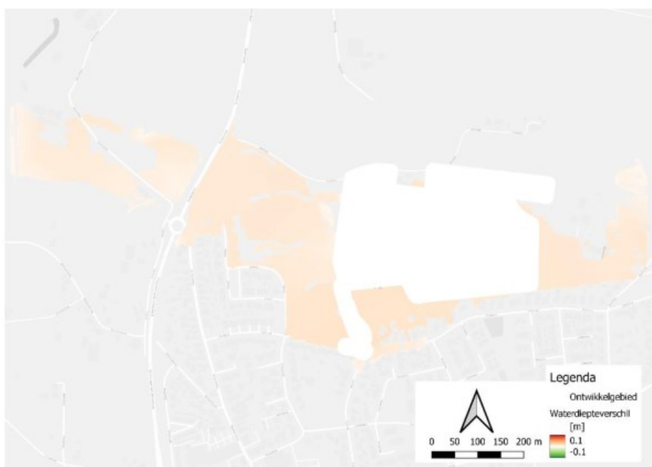
Figuur 4-7 Waterdiepteverschil toekomst situatie t.o.v. bestaande situatie in T1000-scenario. Rood geeft aan waar de maximale waterdiepte toeneemt, groen geeft aan waar de maximale waterdiepte afneemt.
