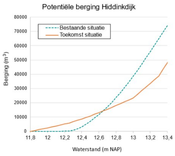
Figuur 4-1 Theoretische bergingscurves bestaande en toekomst situatie Hiddinkdijk
