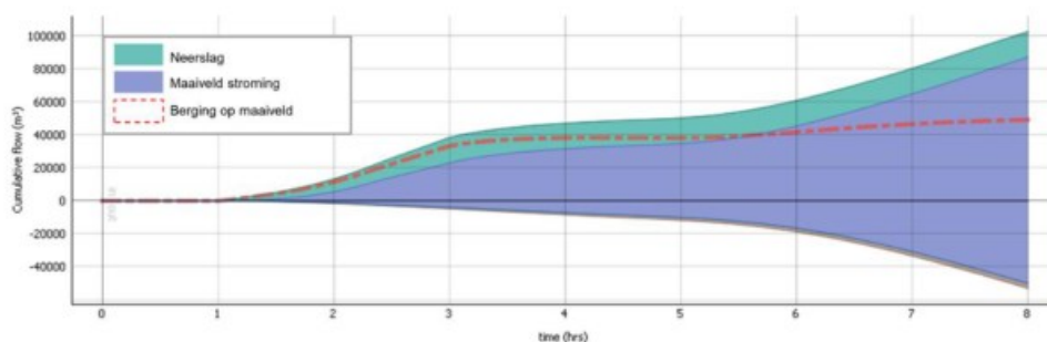
Figuur 3-8 Cumulatieve waterbalans huidige situatie in T1000-scenario
