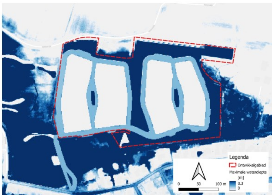
Figuur 4-6 Maximale waterdiepte toekomst situatie in T1000-scenario
