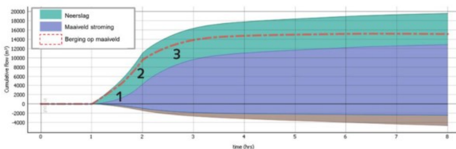
Figuur 3-3 Cumulatieve waterbalans huidige situatie voor het T100-scenario
