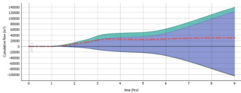
Figuur 4-8 Cumulatieve waterbalans toekomst situatie in T1000-scenario
