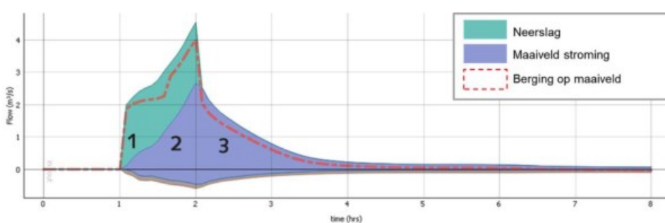
Figuur 3-2 Waterbalans huidige situatie voor het T100-scenario
