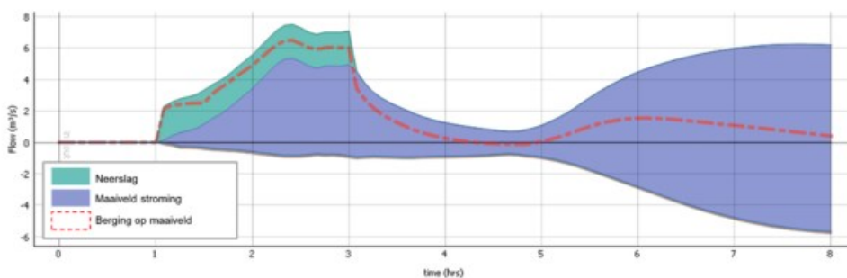
Figuur 3-7 Waterbalans huidige situatie in T1000-scenario
