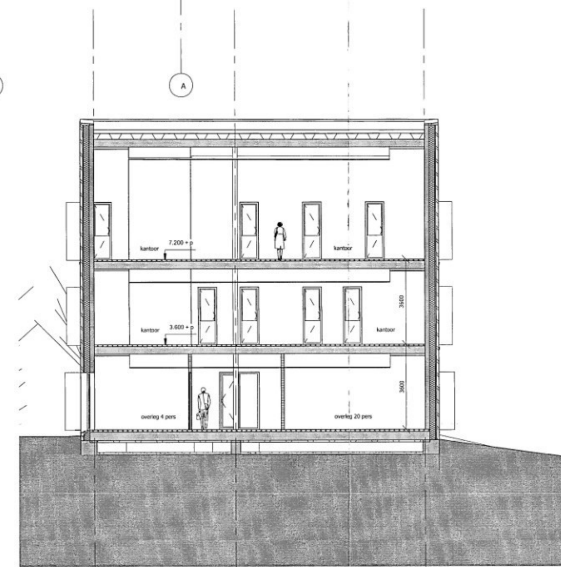
doorsnede DD
