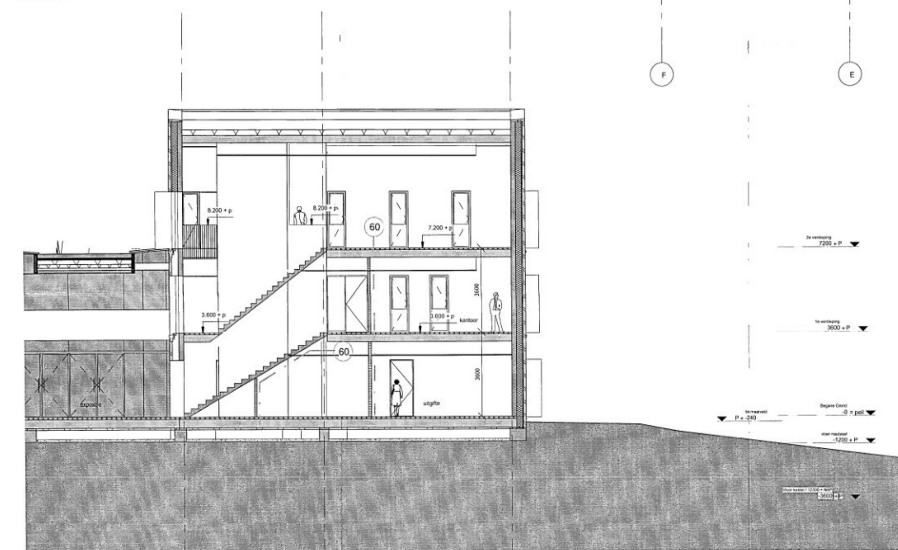
doorsnede CC
