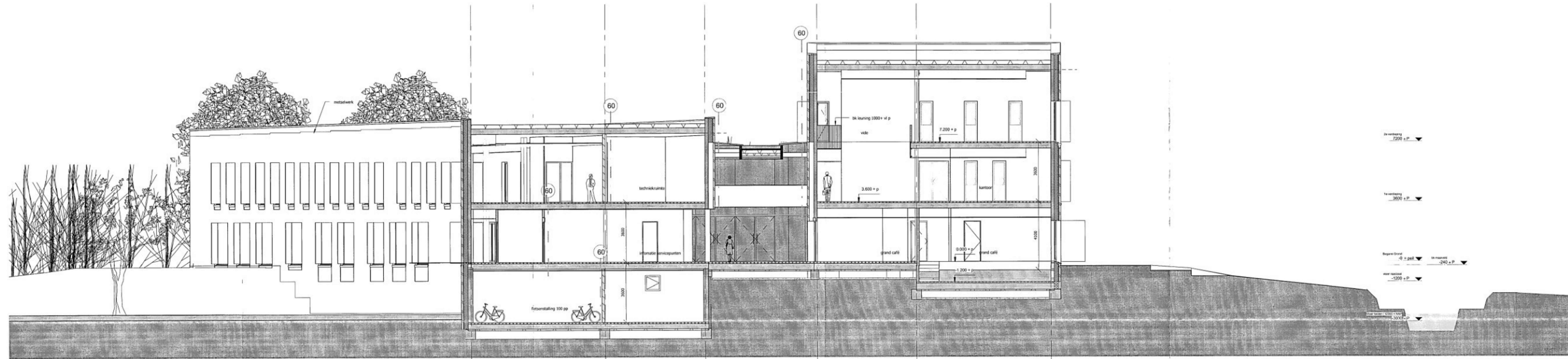
doorsnede BB
