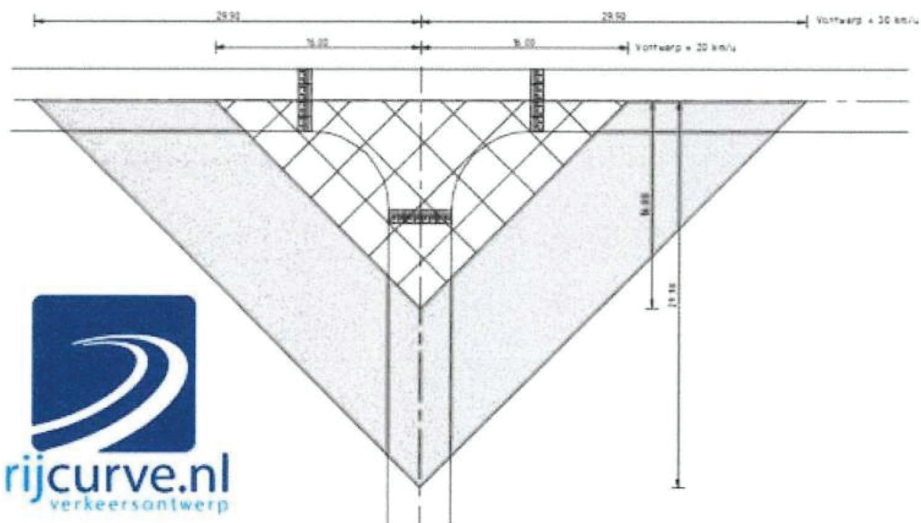
Ideaal situatie bij ontwerpsnelheden 20 km/u en 30 km/u
