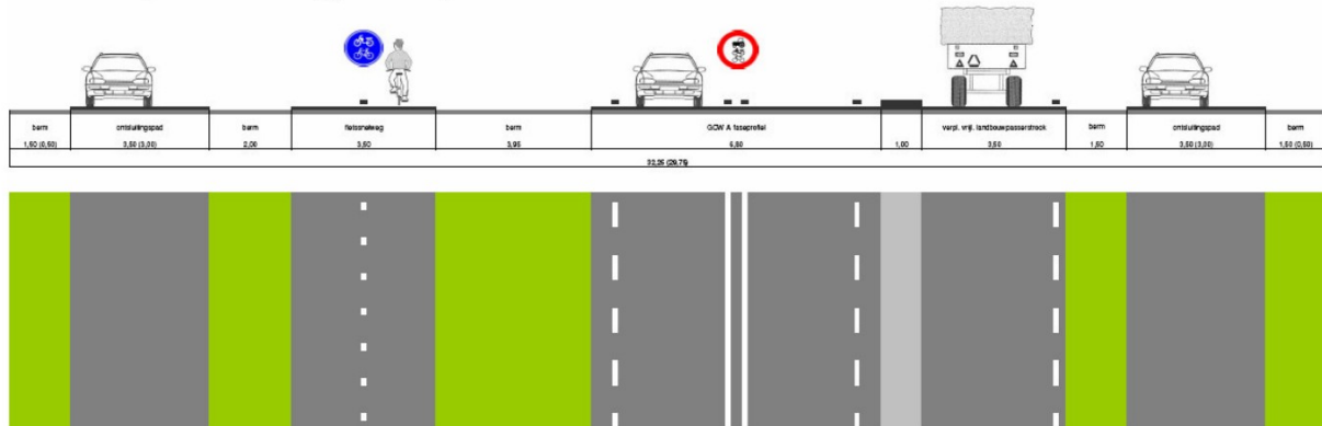
Variant 2b: Landbouwpasseerstroken met ontsluitingspaden aan beide zijden
