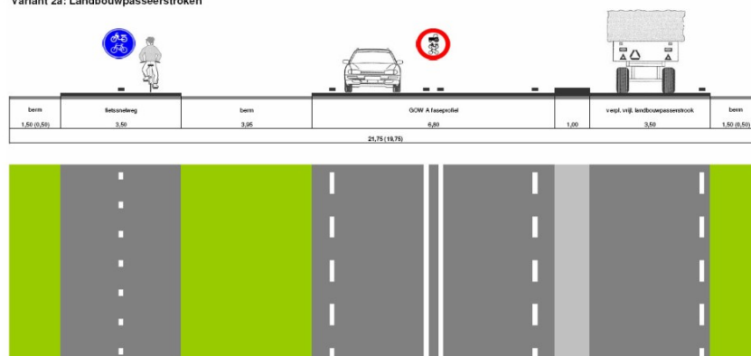
Variant 2a: Landbouwpasseerstroken
