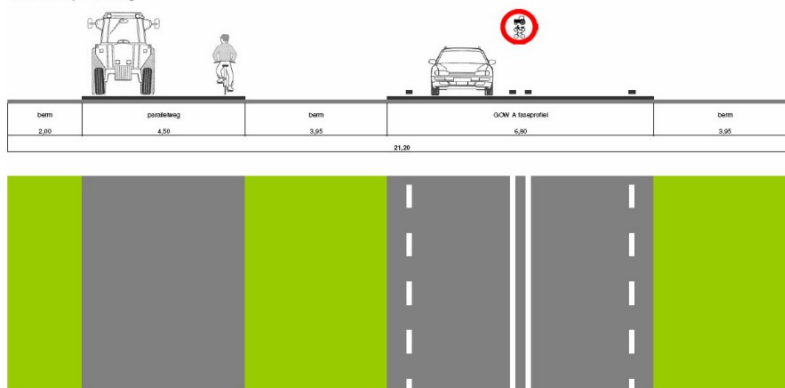
Variant 3a: parallelweg
