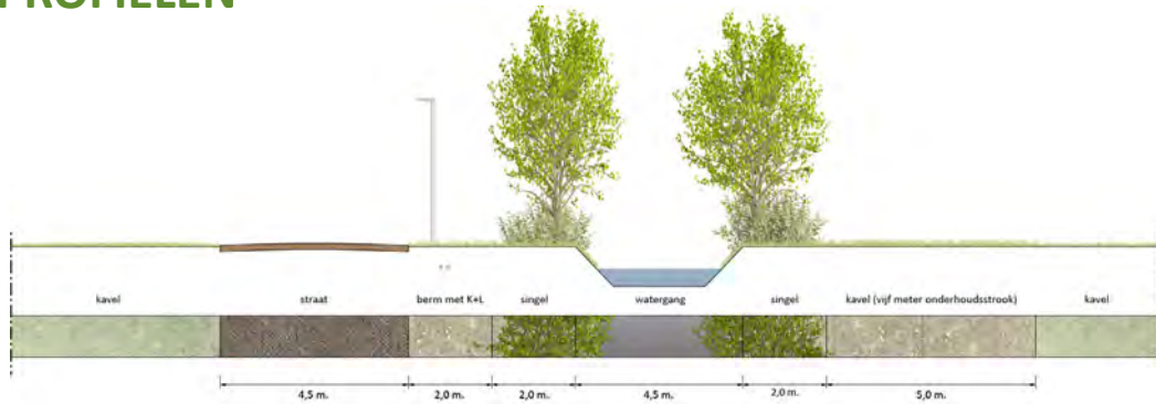
Profiel A-A' - oostelijke deel noordelijke weg
