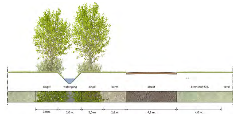
Profiel E-E' - zuidelijke weg
