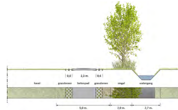
Profiel D-D' - betonpad
