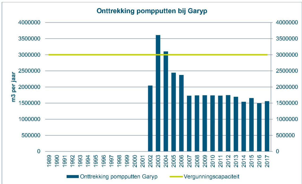
Figuur 2-3 Hoeveelheid werkelijk onttrokken grondwater bij Garyp
