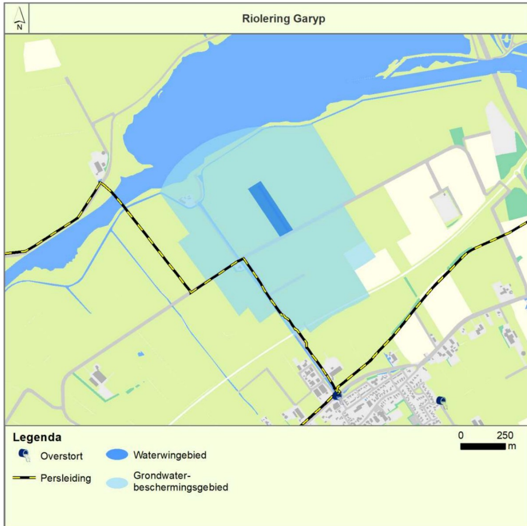
Figuur 6-4 Ligging riolering Garyp
