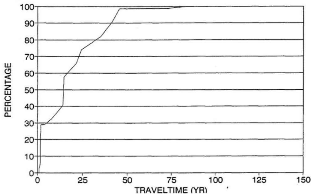
Figuur 4-3 Responsecurve van de winning Ameland Buren (Vitens, 2010)
