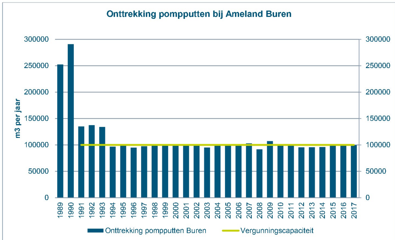
Figuur 2-3 Hoeveelheid werkelijk onttrokken grondwater bij Ameland Buren
