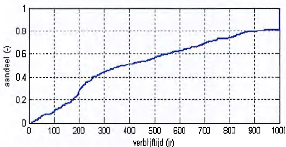
Figuur 4-3 Responscurve van de winning Spannenburg (Vitens, 2010)
