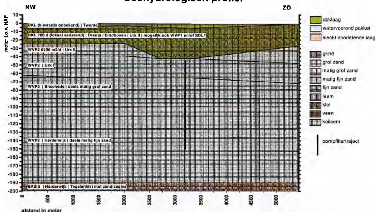
Figuur 4-1 Schematische weergave van de ondergrond ter plaatse van de grondwaterwinning (Bron: Vitens)
