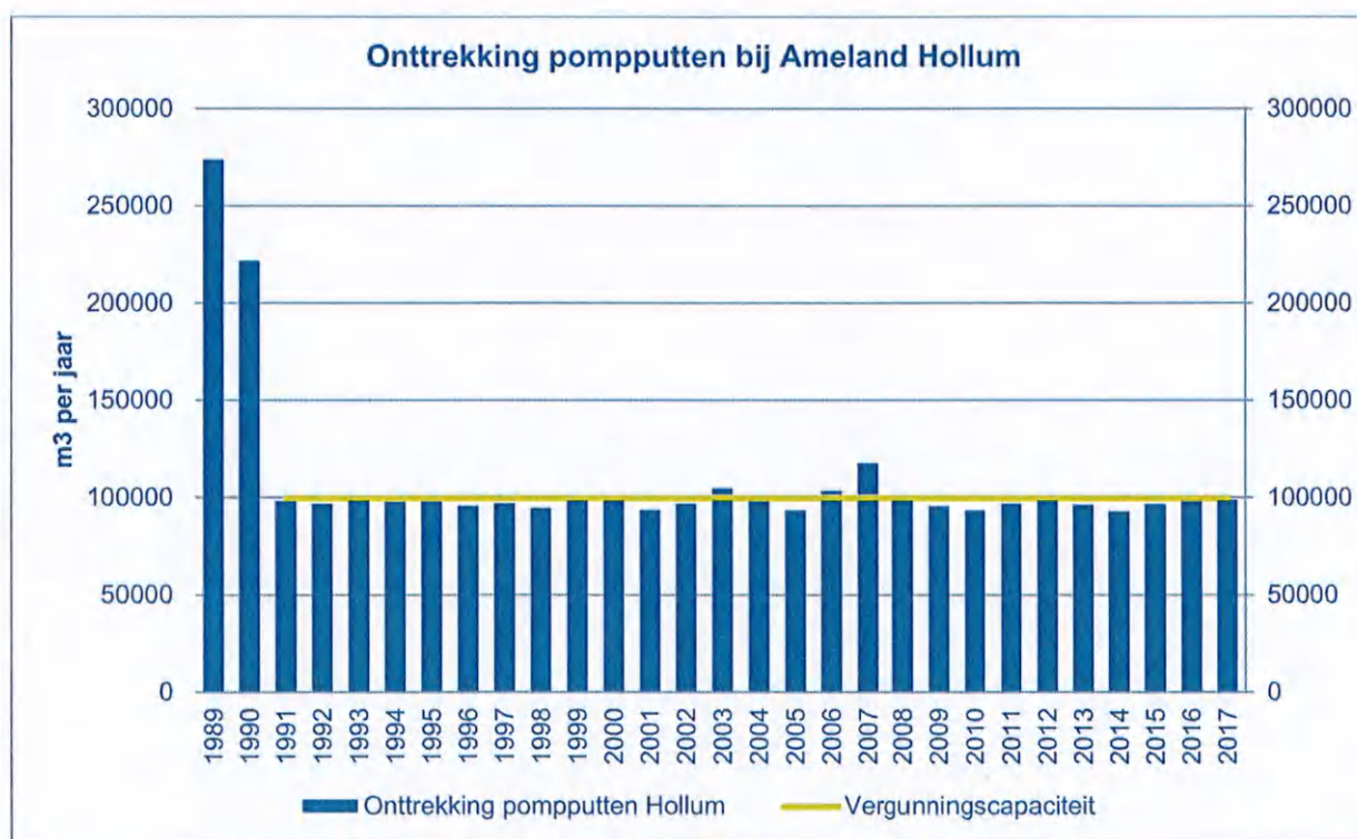
Figuur 2-3 Hoeveelheid werkelijk onttrokken grondwater bij Ameland Hollum
