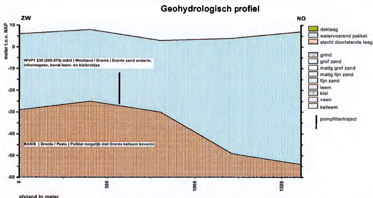
Figuur 4-1 Schematische weergave van de ondergrond ter plaatse van de grondwaterwinning (Bron: Vitens)
