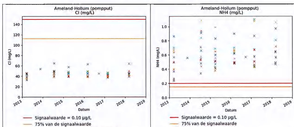
Figuur 5-2 Macroparameters ruw waterkwaliteit
