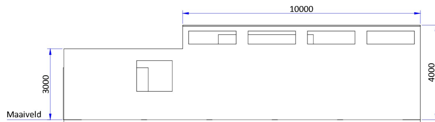
Voor aanzicht (1:100)
