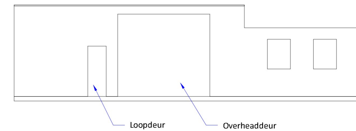
Achter aanzicht (1:100)
