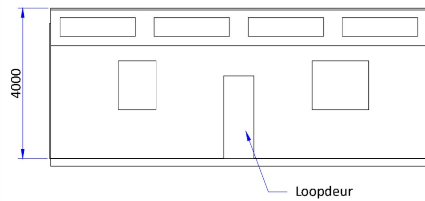
Linker aanzicht (1:100)
