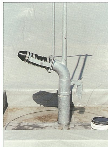
Spuitkop.
