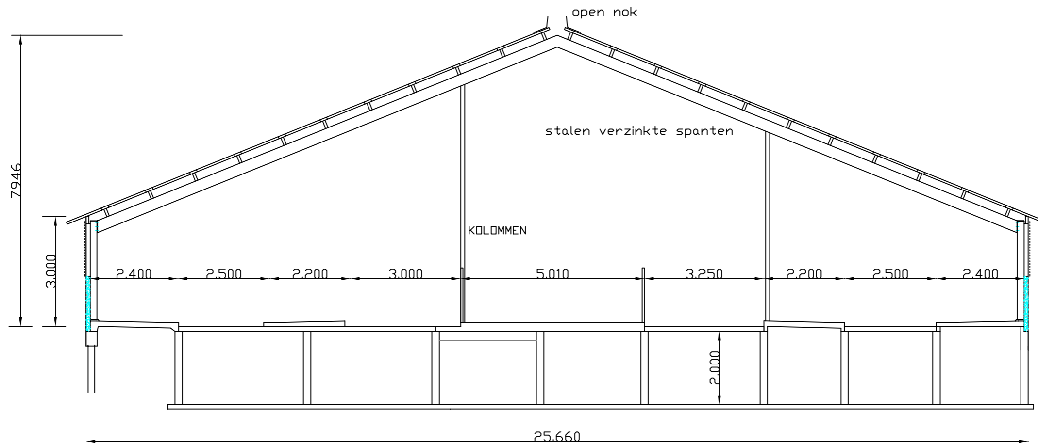
DOORSNEDE STAL
