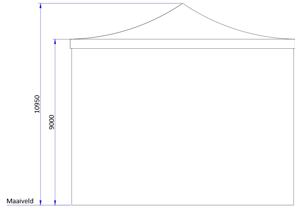
Voor aanzicht (1:100)
