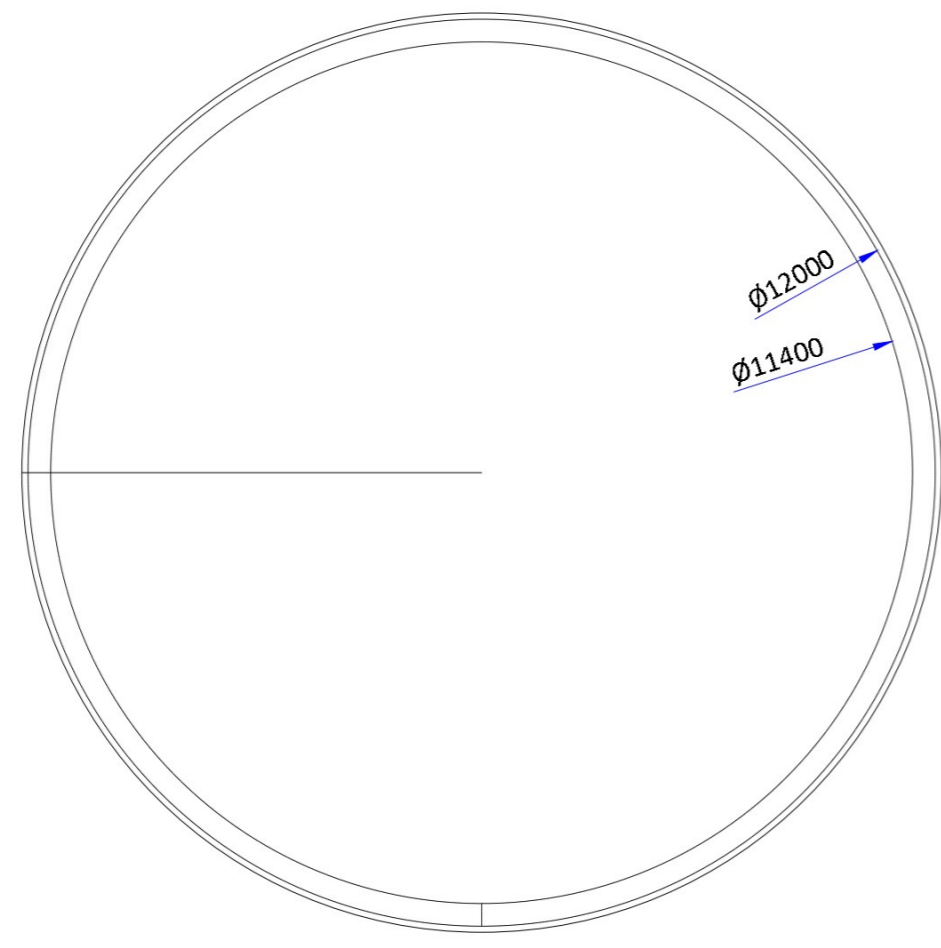
Boven aanzicht (1:100)
