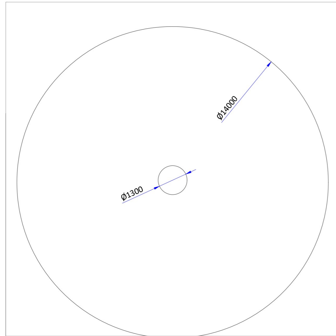
Boven aanzicht (1:100)
