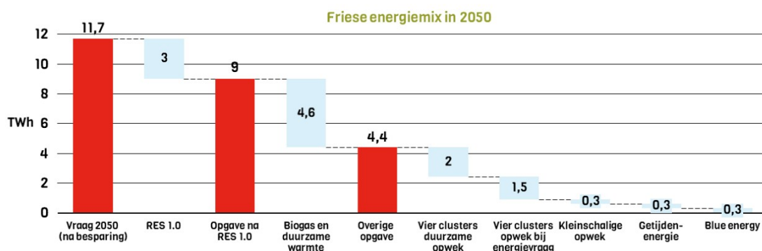
Figuur 3.1 Friese energiemix in 2050, inclusief het RES-bod en invulling van de overige opgave met geclusterde productie van energie, kleinschalige productie en innovatieve technieken.
