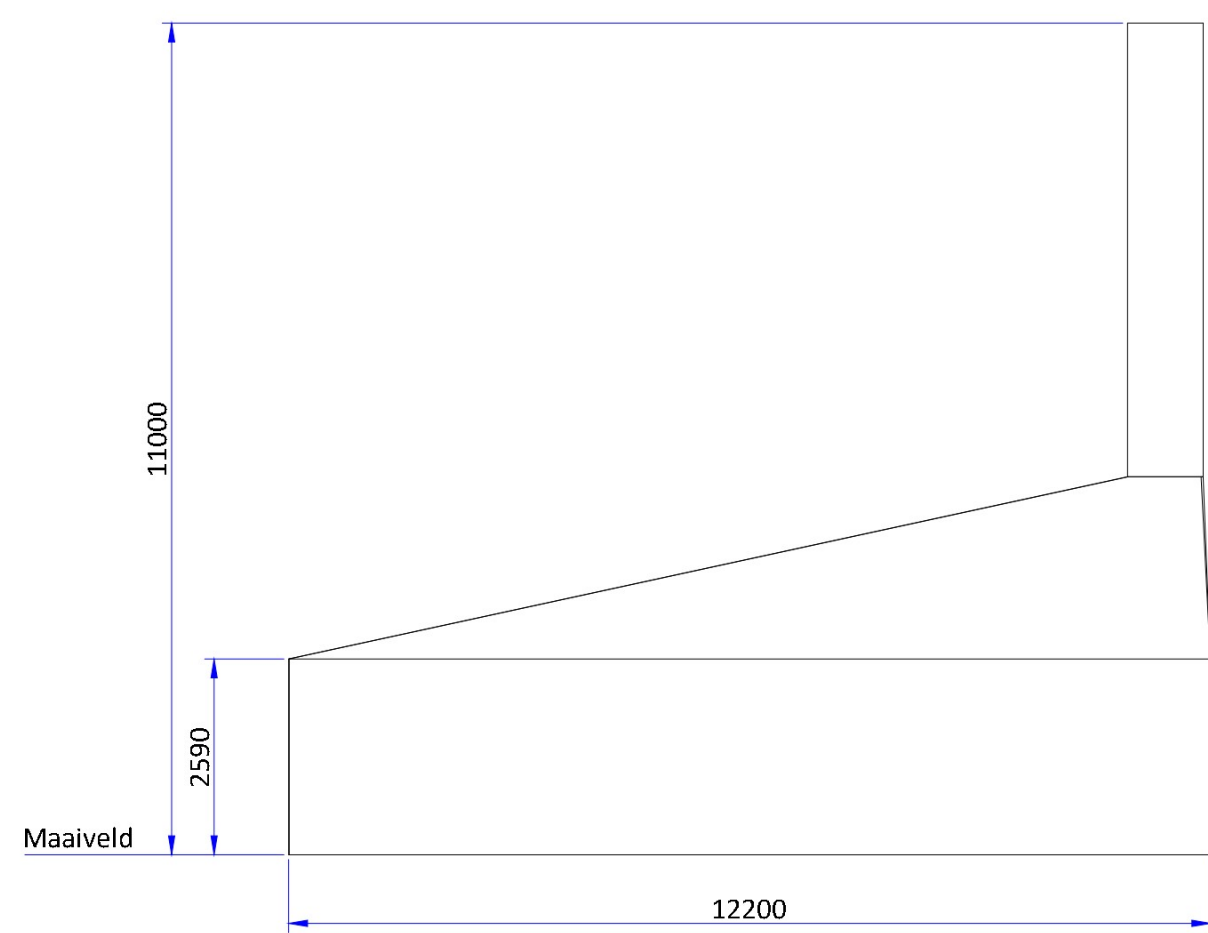
Voor aanzicht (1:100)
