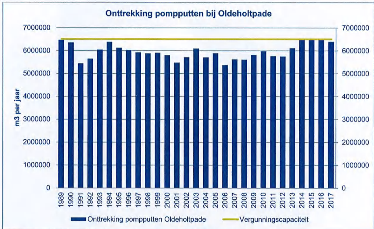
Figuur 2-3 Hoeveelheid werkelijk onttrokken grondwater bij Oldeholtgade
