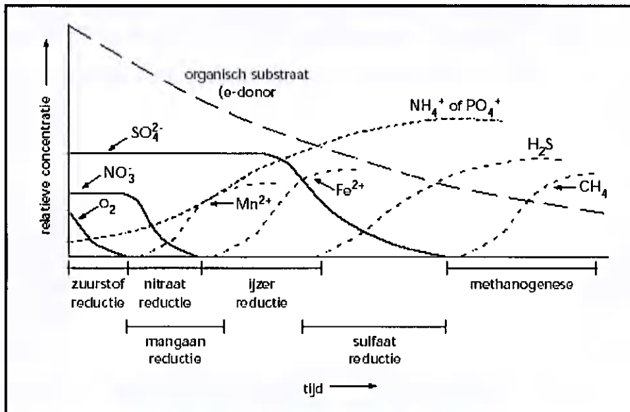
Figuur 4-4 Redox reacties in de ondergrond met toenemende diepte
