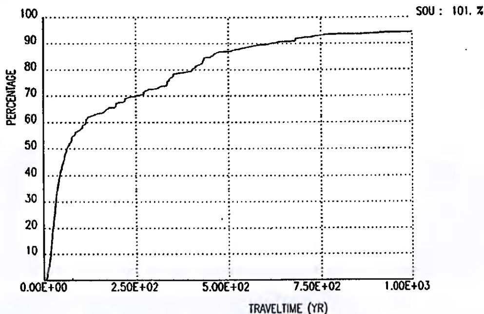
Figuur 4-3 Responscurve van de winning Oldeholtpade (Vitens, 2010)
