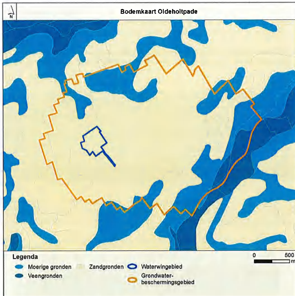
Figuur 4-2 Bodemkaart Oldeholtgade
