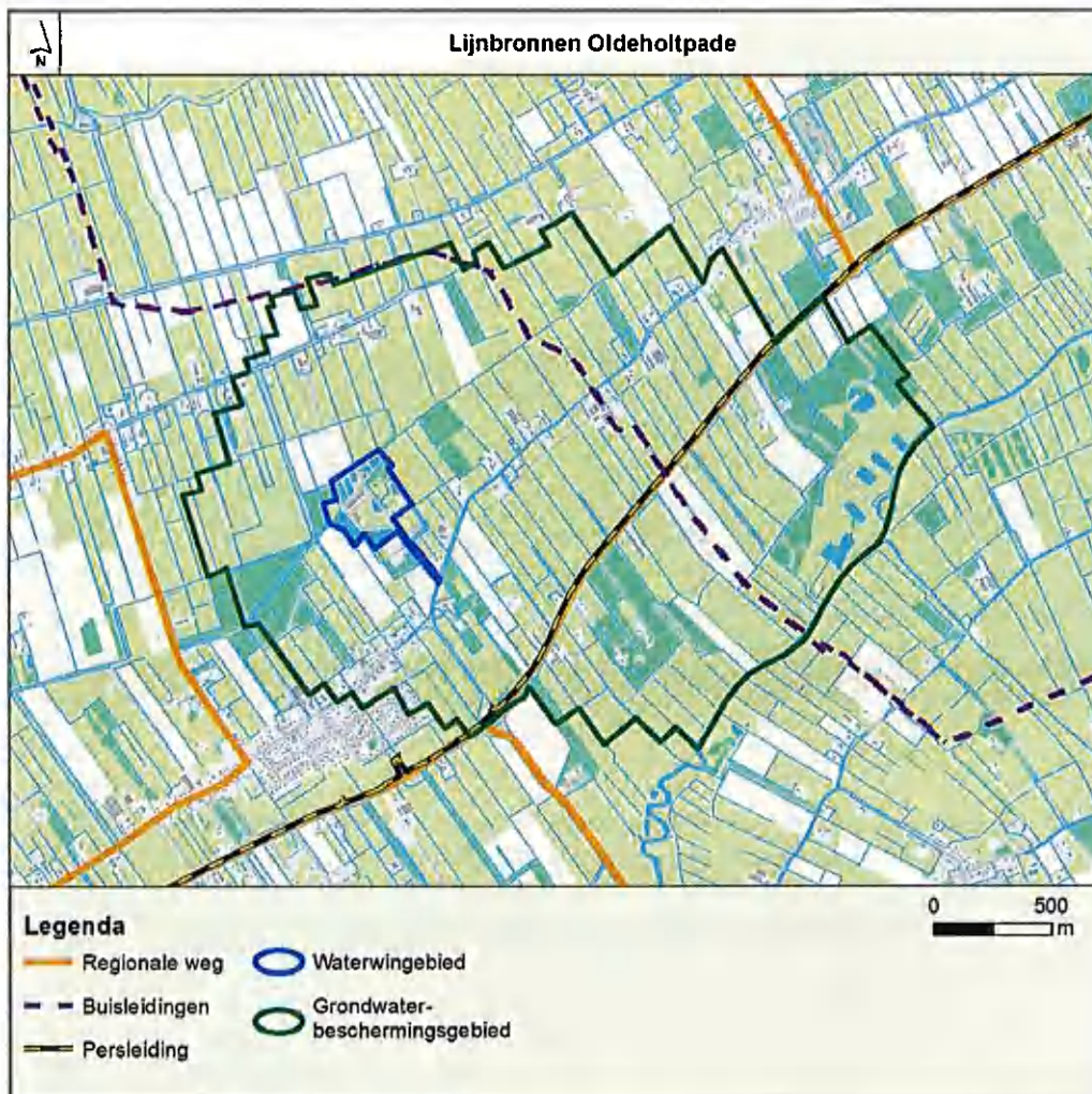
Figuur 6-3 Lijnbronnen Oldeholtpade
